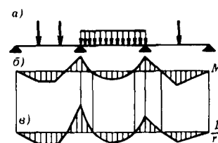
Черт. 21. Эпюры изгибающих моментов и кривизны для железобетонных элементов постоянного сечения а — схема расположения нагрузки; б — эпюра изгибающих моментов; в — эпюра кривизны
