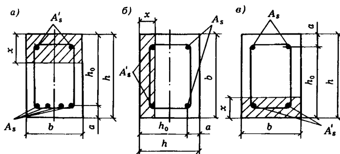
Черт. 14. Схемы расположения сжатой зоны пространственного сечения
