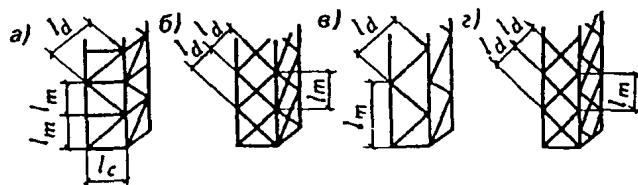
Черт. 8. Схемы пространственных решетчатых конструкций из одиночных уголков
