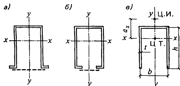
Черт. 2. П-образные сечения элементов
