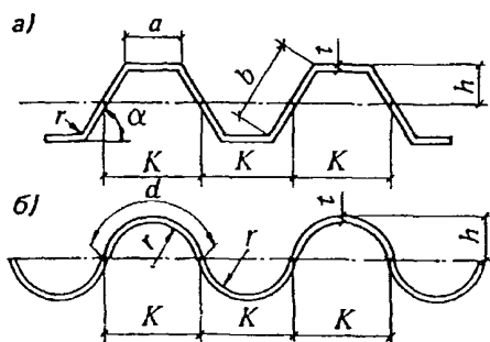
Черт. 13. Геометрические параметры для гофра
