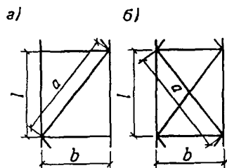
Черт. 3. Схема решетки а — раскосной; б — крестовой с распорками
