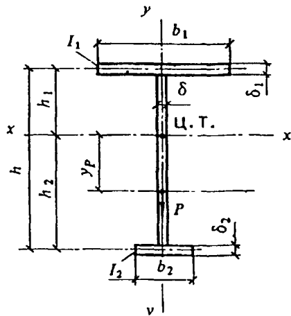
Поперечное сечение балки с развитым верхним поясом
