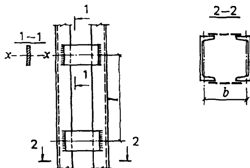
Черт. 4. Составной стержень на планках
