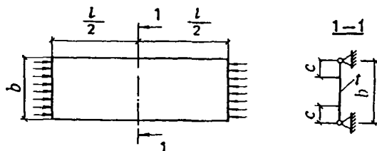
Черт. 10. Расчетная схема сжатого тонколистового элемента
