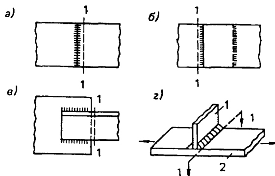
Черт. 1. Схемы сварных соединений конструкций
