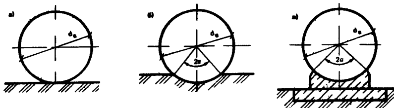
Рис. 2. Способы опирания трубопроводов а — на плоское грунтовое основание; б — на грунтовое профилированное основание с углом охвата 2\alpha ; в — на бетонный фундамент
