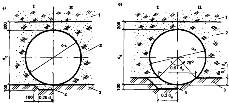
Рис. 1. Способы опирания труб на основание а — плоское грунтовое основание; б — профилированное грунтовое основание с углом охвата 75^\circ ; 1 — с песчаной подушкой; II — без песчаной подушки; I — засыпка местным грунтом без уплотнения; 2 — засыпка местным грунтом с нормальной или повышенной степенью уплотнения; 3 — естественный грунт; 4 — подушка из песчаного грунта
