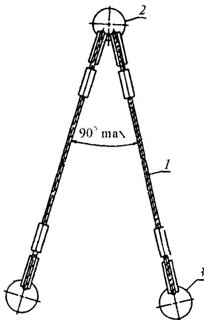
Рис. П.1.22. Двухветевой строп: 1 — канатная ветвь, 2 — звено, 3 — захват
