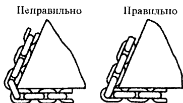
Рис. П.3.2. Строповка грузов цепными стропами
