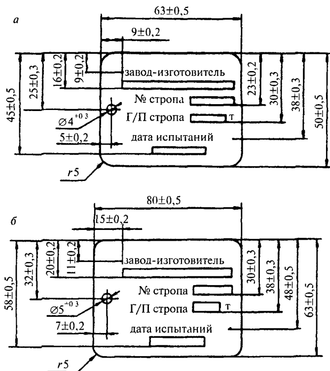
Рис. П.2.1. Бирки маркировочные: а — для стропов грузоподъемностью до 3,2 т; б — свыше 3,2 т
