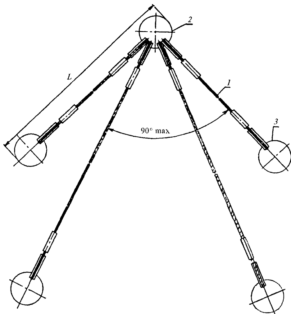
Рис. П.1.24. Четырехветевой строп: 1 — канатная ветвь, 2 — звено, 3 — захват
