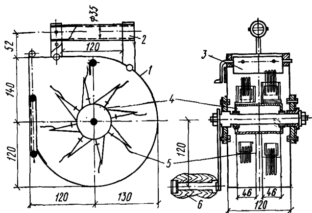
Рис. 7. Приспособление для набрызга декоративного раствора
