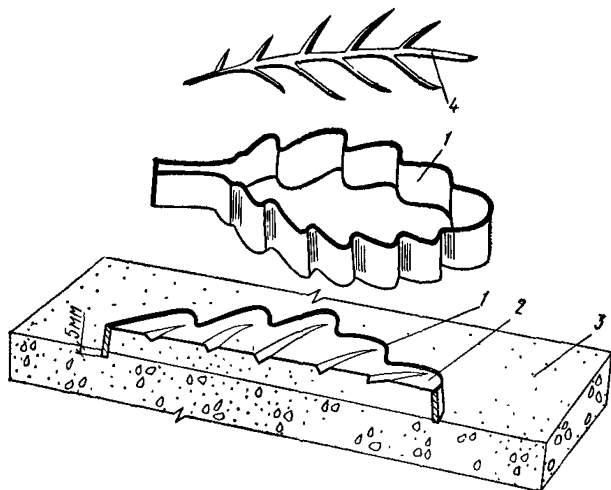
Рис. 3. Контурные шаблоны для укладки цветного раствора
