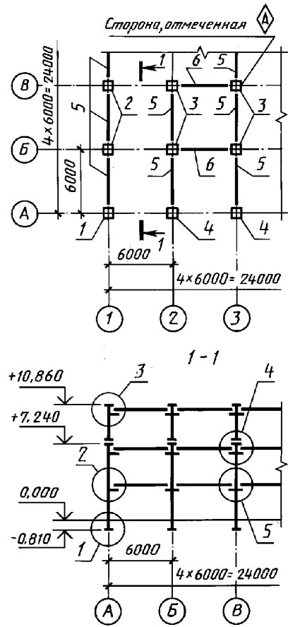
Схема расположения колонн, ригелей и балок перекрытия на отм...
