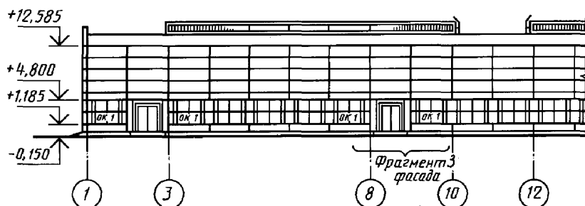
Фрагмент 3 фасада
