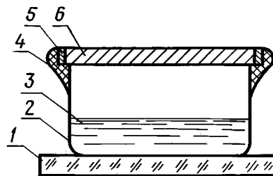
Схема прибора для определения сопротивления паропрооницаемости
