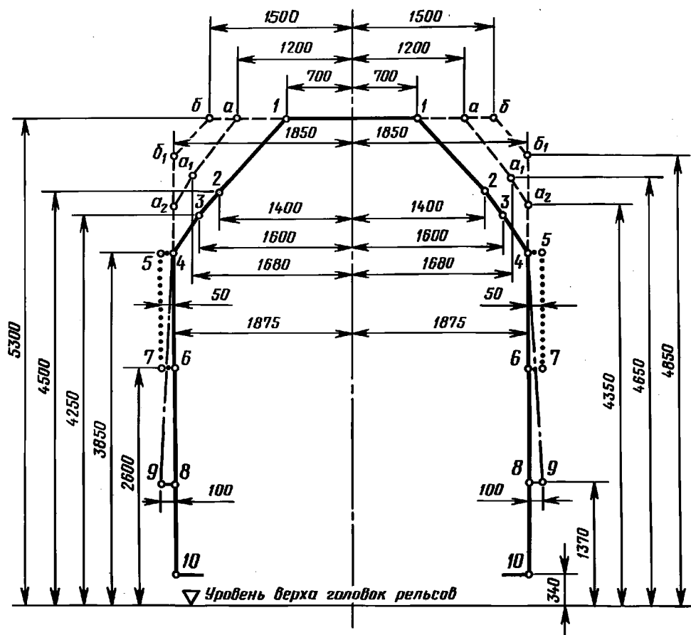
Габарит Т Верхнее очертание габарита
