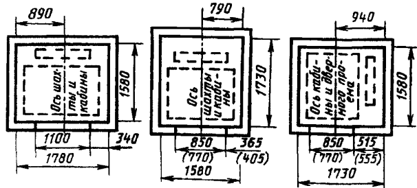
Противовес сзади кабины
