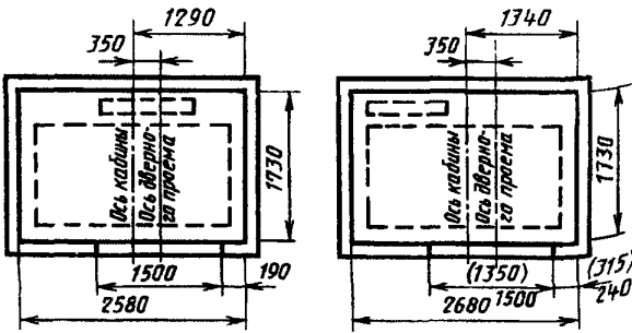
Противовес сзади кабины
