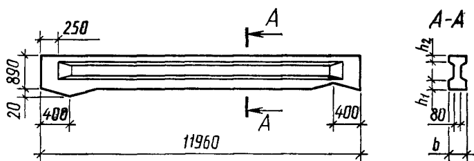
Черт. 9
