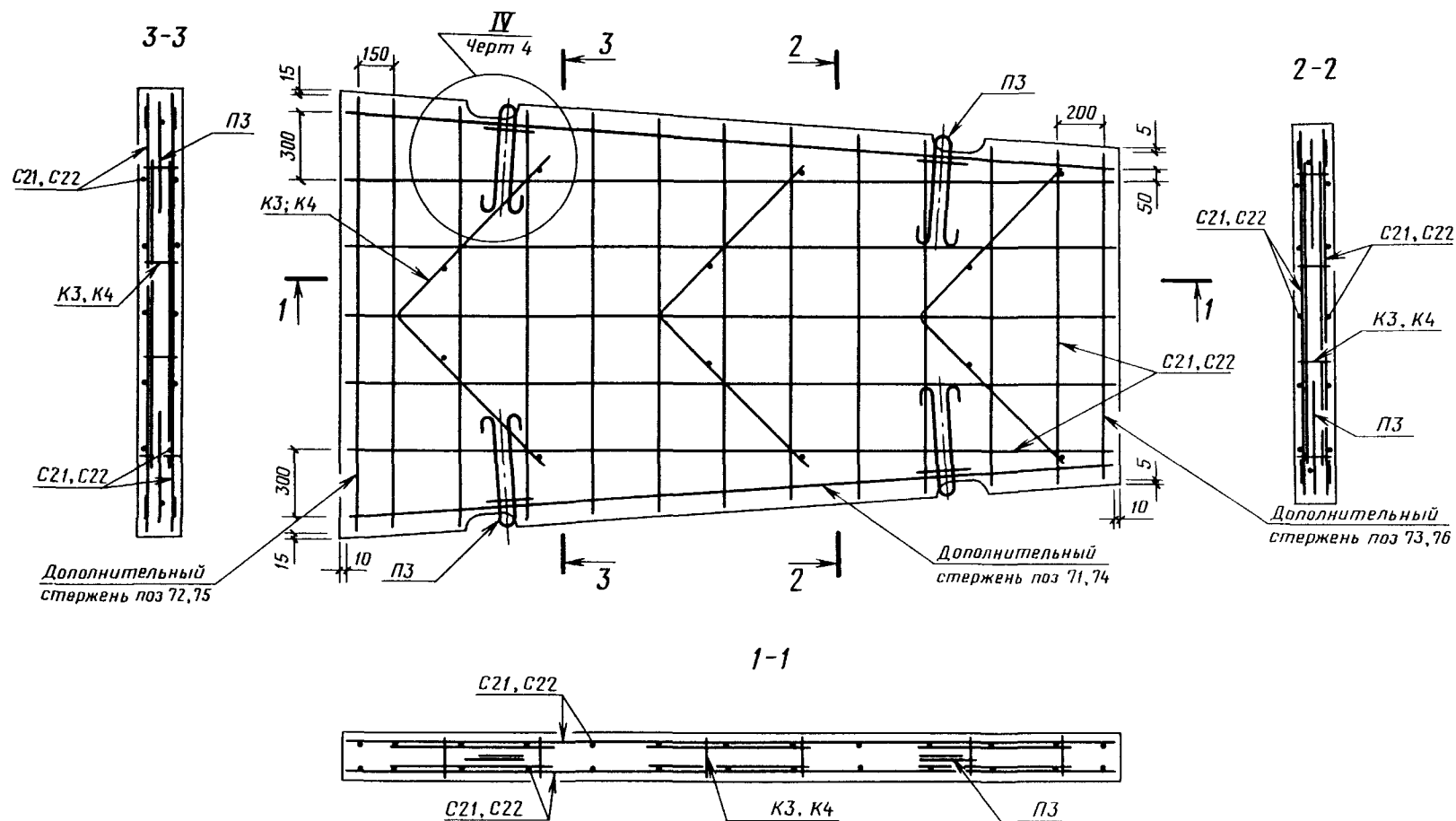
Плита ПТ35
