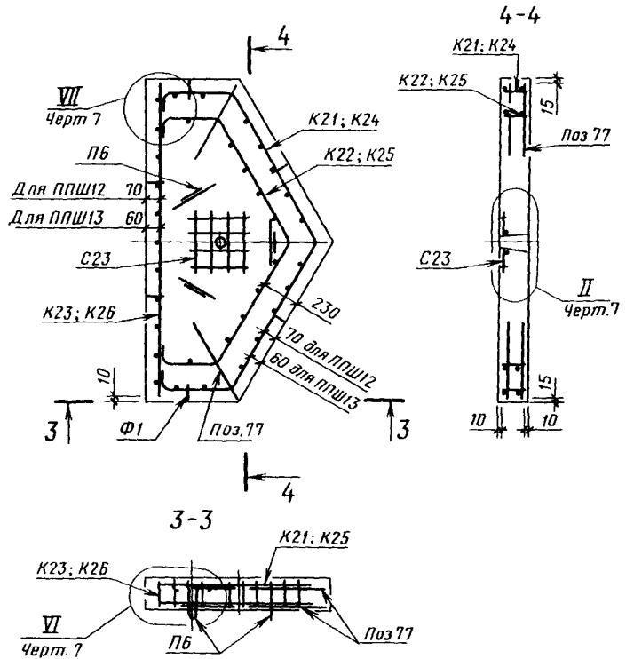
Плиты ППШ13 и ППШ12
