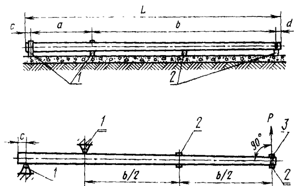
Схема испытания стоек
