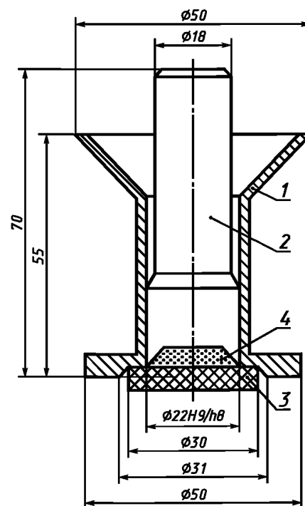
Воронка с пуансоном
