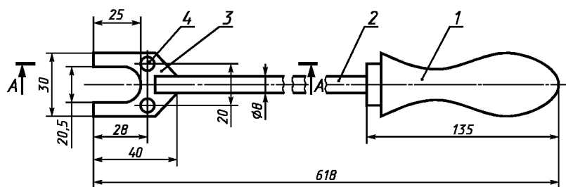
A-A (2:1)
