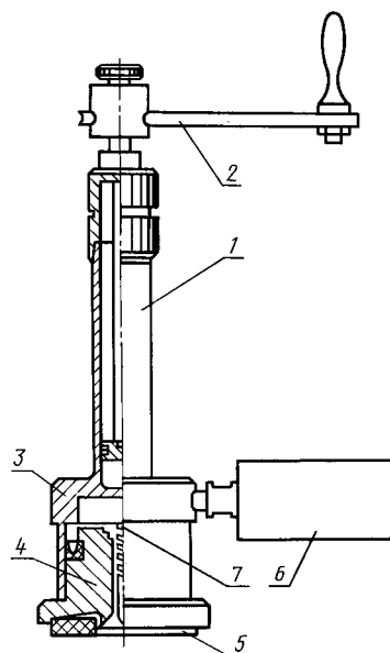
Филтратометр ФМ-3
