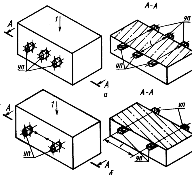
a — схема испытания призм способом сквозного прозвучивания; b — схема испытания призм способом поверхностного прозвучивания; УП — ультразвуковые преобразователи; I — направление формования
