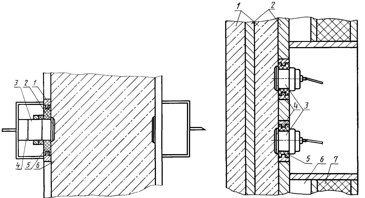
1 — бетон; 2 — разделительные листы кассеты; 3 — преобразователи; 4 — рабочие поверхности преобразователей; 5 — акустическая изоляция; 6 — паровая рубашка; 7 — теплоизоляция
