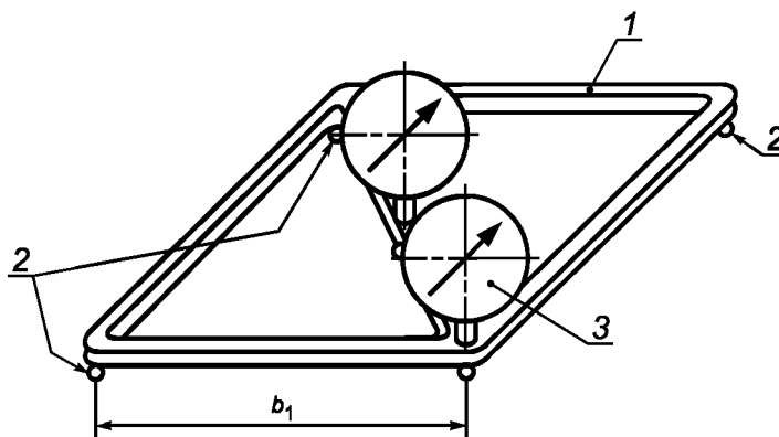
Схема прибора для измерения отклонений от плоскостности
