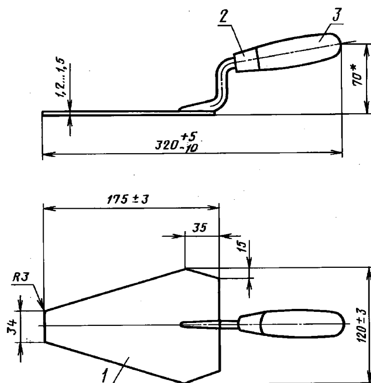
Лопатка типа ЛП
