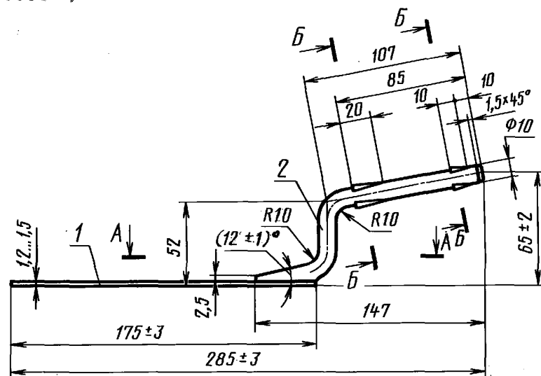
Полотно с кронштейном кельмы типа ЛП
