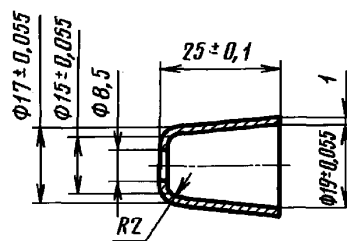
Колпачок для отрезовки
