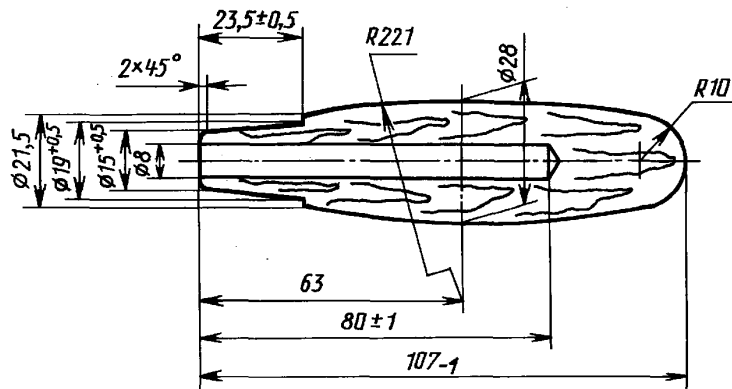
Ручка для отрезовки
