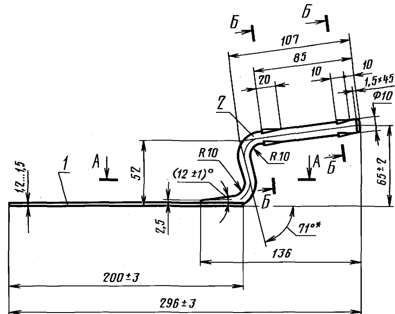
Полотно с кронштейном лопатки типа ЛК
