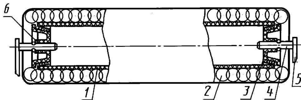
Ролик валика типа ВМП
