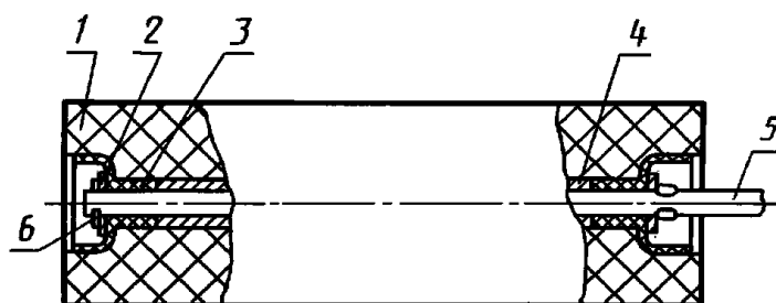
Ролик валика типа ВП
