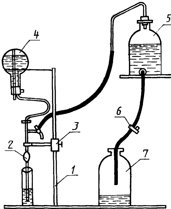
1 — штатив; 2 — пипетка вместимостью 25 \text{ см}^3 ; 3 — упор; 4 — колба для промывания пипетки; 5 — аспириатор; 6 — зажим; 7 — водослив
