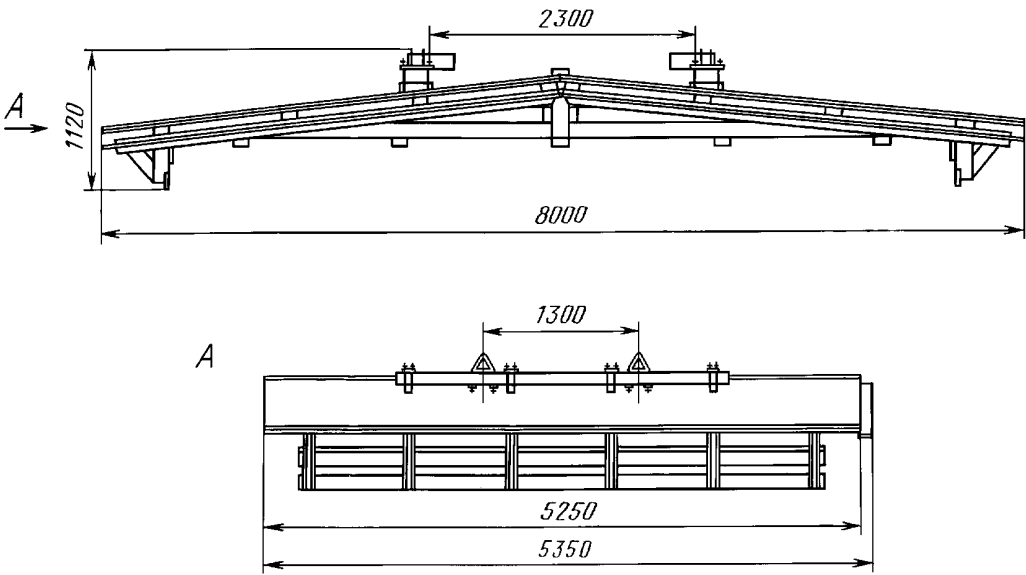
Съемная крыша при формировании штабеля краном
