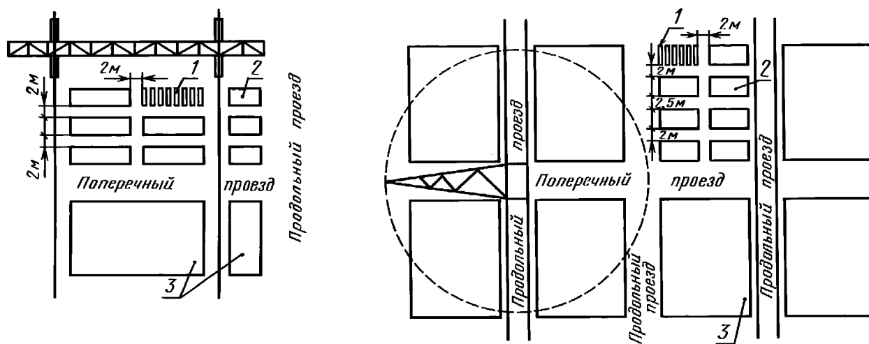
а — КОЗЛОВЫМ
