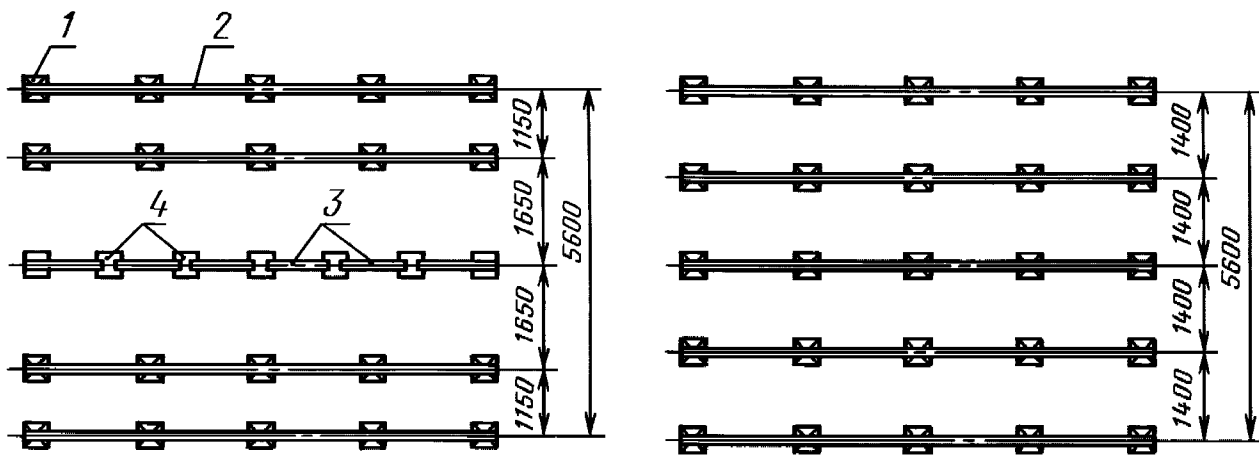
а — автопогрузчиком
