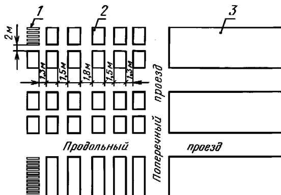
Планировка групп штабелей при пакетной укладке автопогрузчиком
