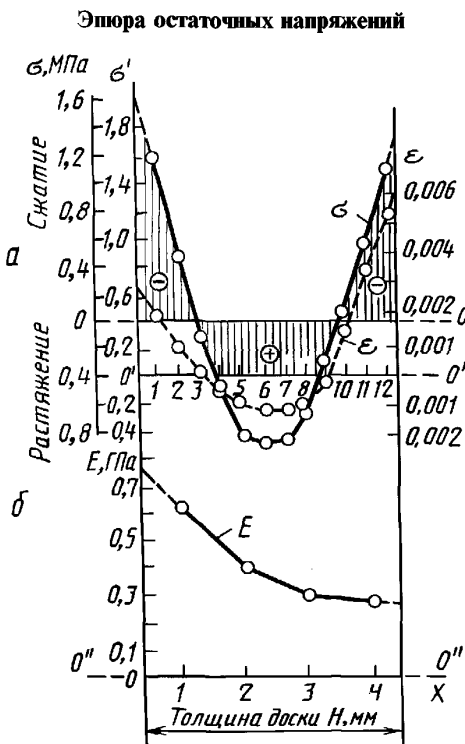
а — кривые напряжений \sigma и деформаций \varepsilon ; б — кривая модуля упругости E .
