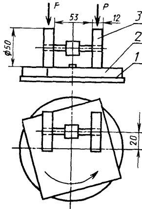
1—поворотный стол 2—образец; 3—фрикционный ролик
