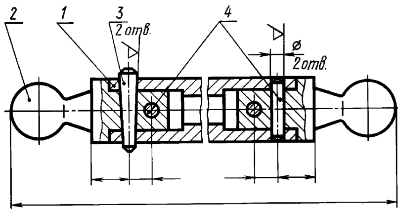
Сборочный чертеж
