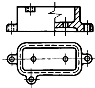
Черт. 24
