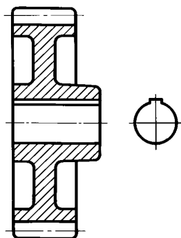
Черт. 60
