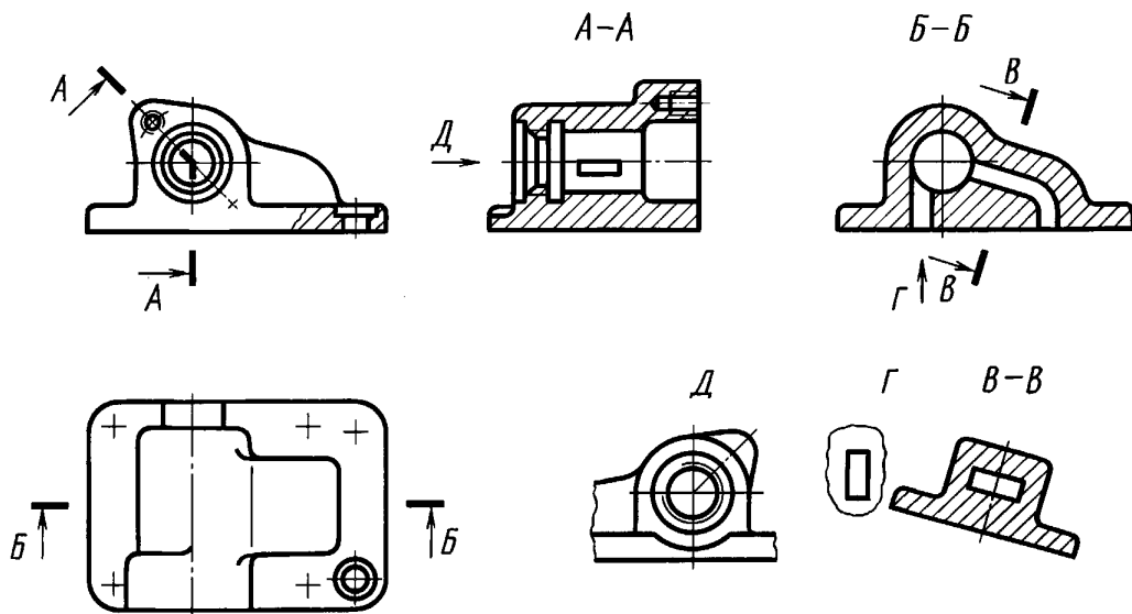
Черт. 8
