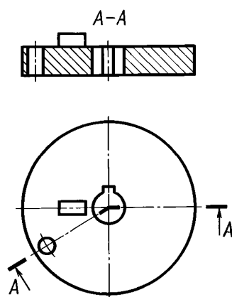
Черт. 20
