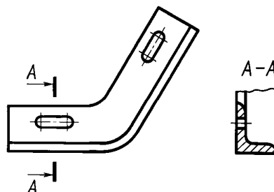
Черт. 38
