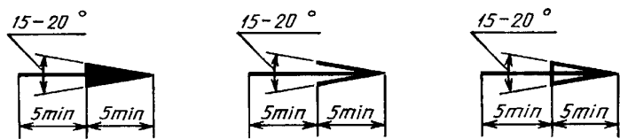
Черт. 14
