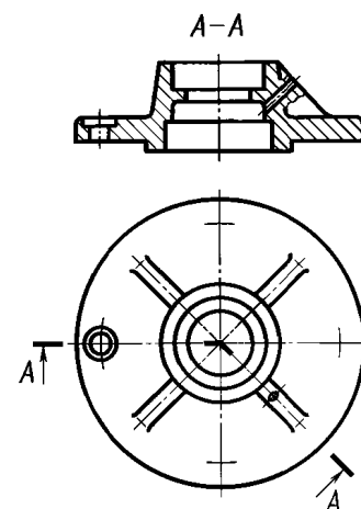
Черт. 53
