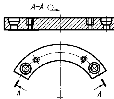
Черт. 7
