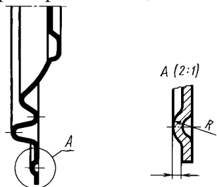
Черт. 39
