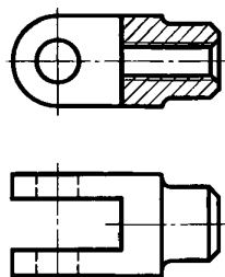
Черт. 4
