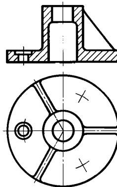
Черт. 5
