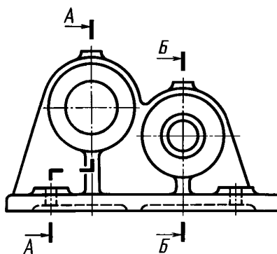
Черт. 61
