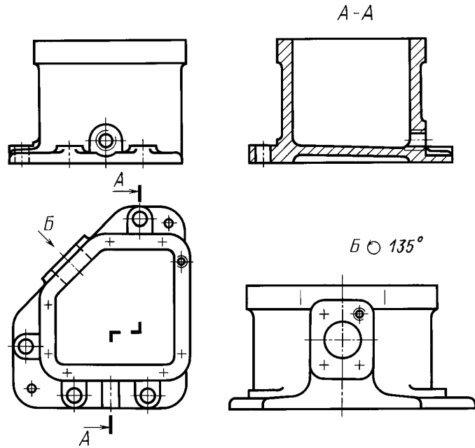
Черт. 12
