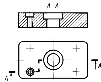
Черт. 16
