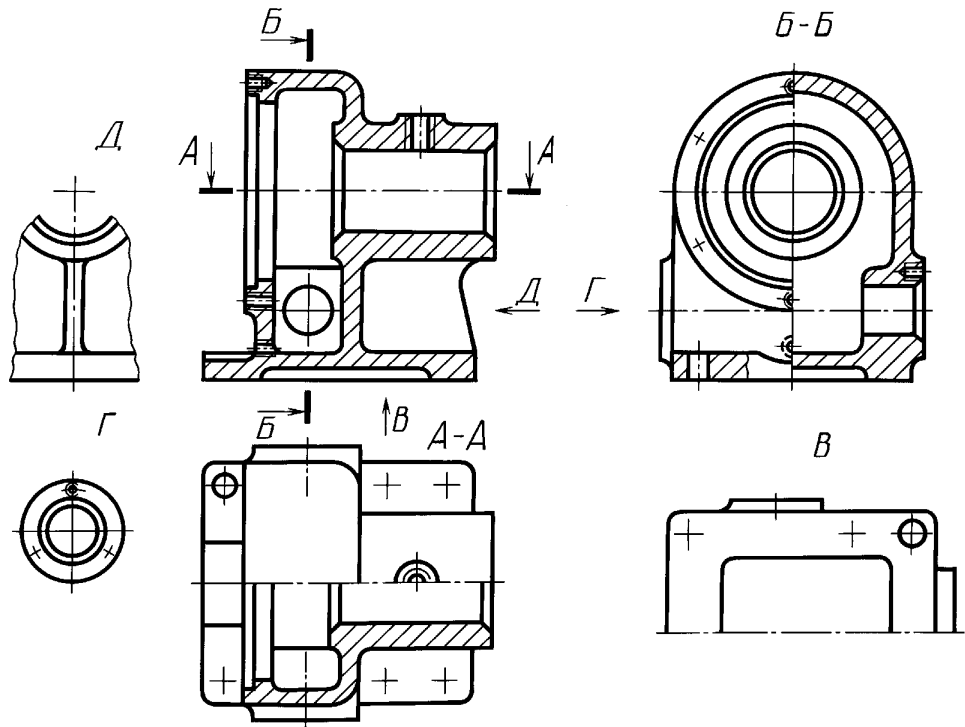
Черт. 13
