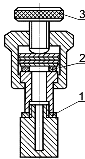
1 — металлическая прокладка; 2 — испытуемый образец; 3 — зажимной винт
