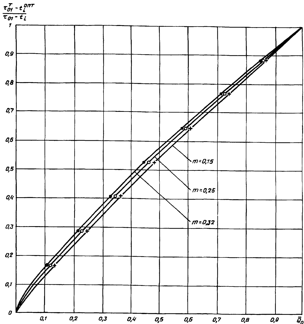
Рис. 2. Графики изменения температурного критерия системы отопления по температуре воды в подающем трубопроводе \frac{\tau_{01}^T - t_i^{\text{опт}}}{\tau_{01} - t_i} для различных значений показателя степени m и при постоянной циркуляции теплоносителя в системе
