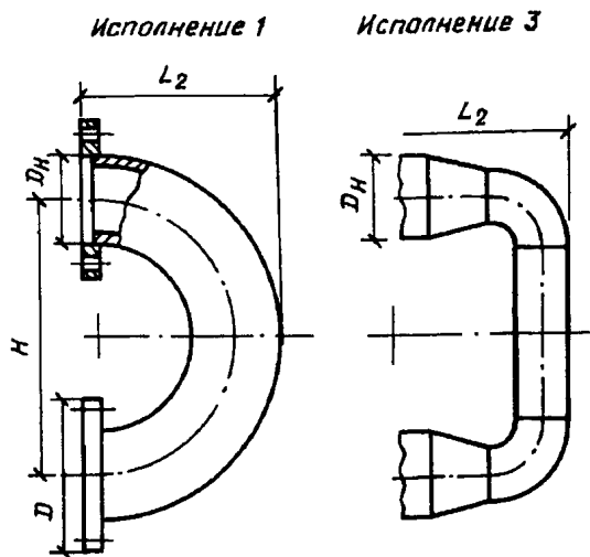
Рис. 3. Калач соединительный
