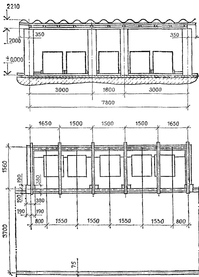
Рис. 20. Площадка крытая для пяти контейнеров
