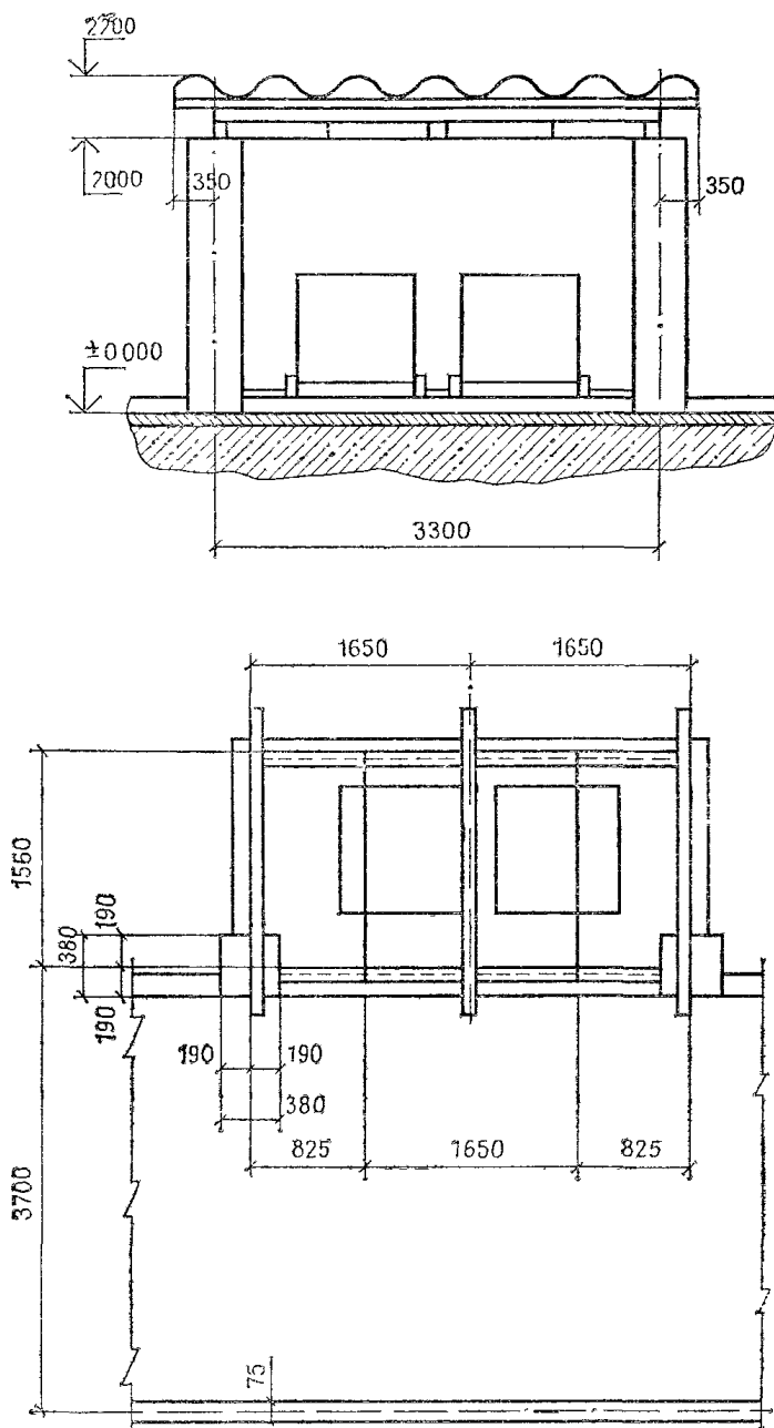
Рис. 19. Площадка крытая для двух контейнеров
