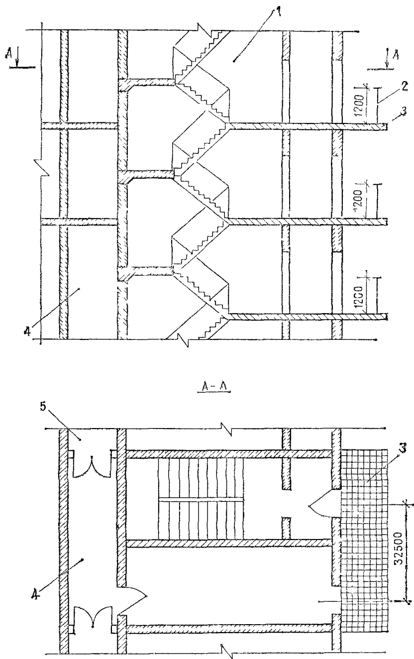
Рис. 24. Пример планировочного решения лестничной класки с переходом через наружную воздушную зону по балконам
