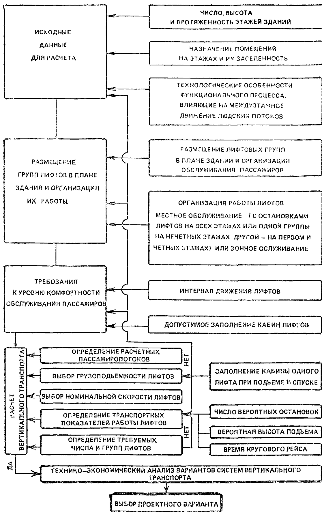
Блок-схема расчета вертикального транспорта
