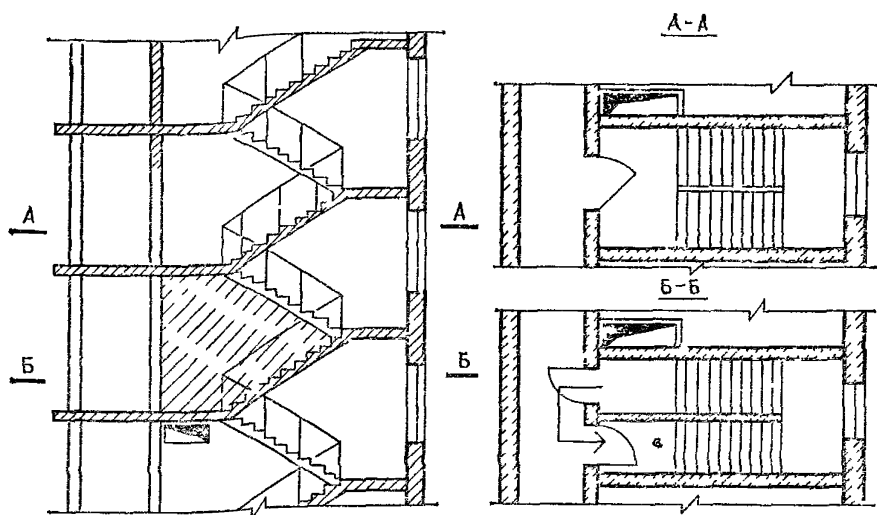
Рис. 25 Устройство расщепки между тарсами в лестничной клетке с подпором воздуха
