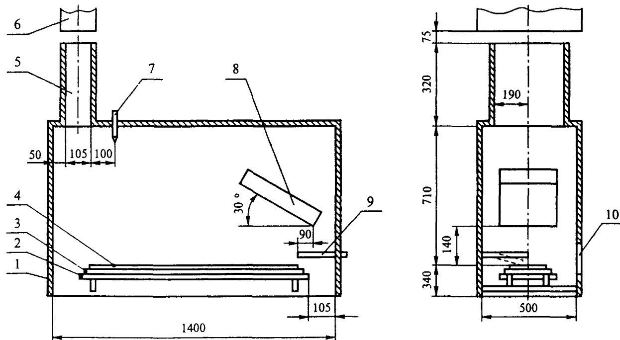
1 — испытательная камера; 2 — платформа; 3 — держатель образца; 4 — образец; 5 — дымоход; 6 — вытяжной зонт; 7 — термopapa; 8 — радиационная панель; 9 — газовая горелка; 10 — дверца со смотровым окном
