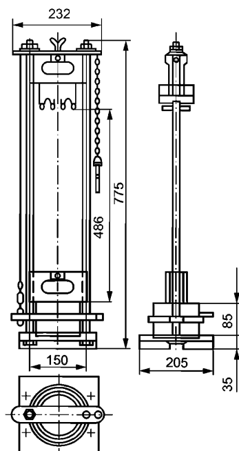
Рисунок 7 — Копер ПМ
