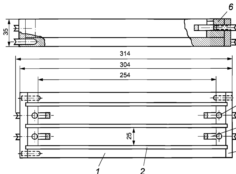
1 — форма; 2 — боковые стенки формы; 3 — торцевая стенка формы; 4 — репер; 5 — стопорный винт для крепления репера; 6 — держатель репера
