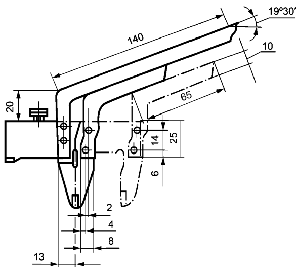
Рисунок 3 — Передвижной шаблон
