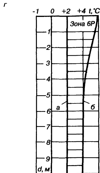
Рисунок А.7 — Эпюры распределения расчетных температур грунта основания по глубине в пределах следующих зон граничных условий: а—6М; б—21; в—6А (1), 6Б (1), 6В (1), 6А (2), 6Б (2), 6В (2); г—6Р
