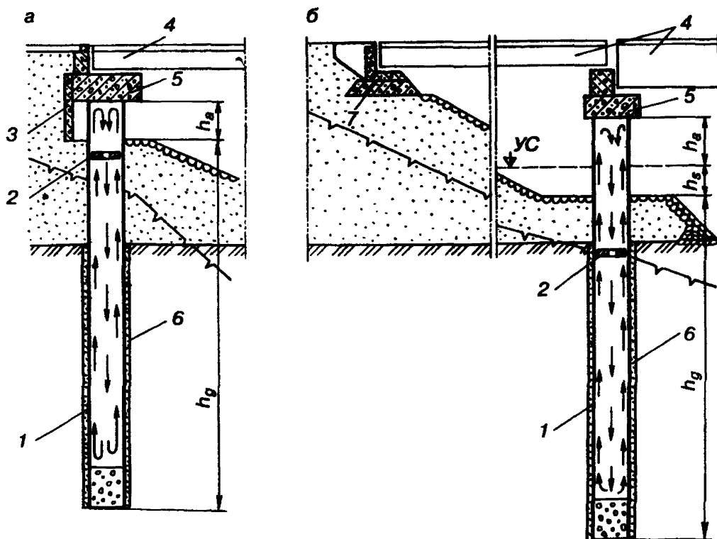
Рисунок Г.1 — Опора со стойками из термоэлементов:
