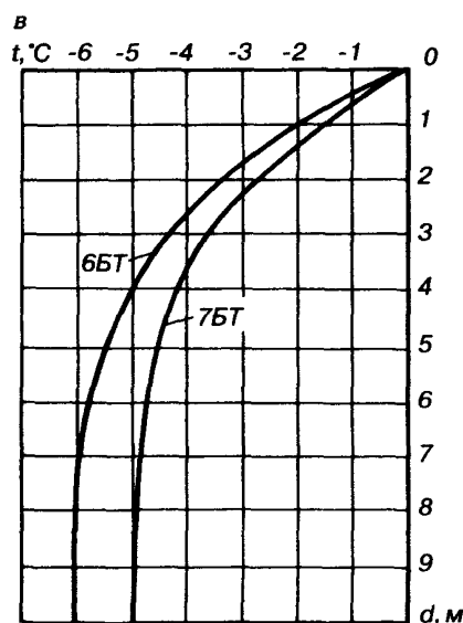
Рисунок А.6 — Эпюры распределения расчетных температур грунта основания по глубине в пределах следующих зон граничных условий: а — 6БП, 7БП, 6Б (3, 4), 6В (3), 7Б, 7В; б — 5БП, 4БП, 4Б (3, 4), 4БМ, 4В (3); в — 6БТ, 7БТ; г — 4БТ, 5БТ, 5А, 5Б, 5В, 4Б (2), 4В (2), 4Б (1), 4В (1)
