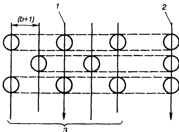
Рисунок Е.1 — Схема к определению коэффициента k при шахматном расположении столбов:
