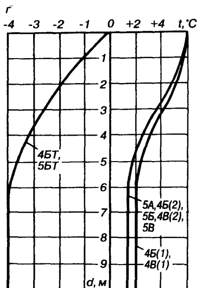
Рисунок А.6 — Эпюры распределения расчетных температур грунта основания по глубине в пределах следующих зон граничных условий: а — 6БП, 7БП, 6Б (3, 4), 6В (3), 7Б, 7В; б — 5БП, 4БП, 4Б (3, 4), 4БМ, 4В (3); в — 6БТ, 7БТ; г — 4БТ, 5БТ, 5А, 5Б, 5В, 4Б (2), 4В (2), 4Б (1), 4В (1)
