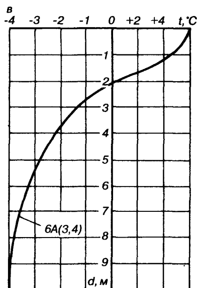
Рисунок А.8 — Эпюры распределения расчетных температур грунта основания по глубине в пределах следующих зон граничных условий: а—1А, 2А (1:1,5), 2А (1:3), 8А (б); б—2А (1:5), 3А (1:5), 3А (1:1,5), 3А (1:3), 8А (а); в—6А (3,4); г—5Г, 12П
