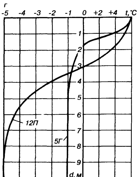
Рисунок А.8 — Эпюры распределения расчетных температур грунта основания по глубине в пределах следующих зон граничных условий: а—1А, 2А (1:1,5), 2А (1:3), 8А (б); б—2А (1:5), 3А (1:5), 3А (1:1,5), 3А (1:3), 8А (а); в—6А (3,4); г—5Г, 12П
