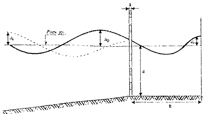
Рисунок 6.3 - Взаимодействие волн с пропускаемым сооружением:
