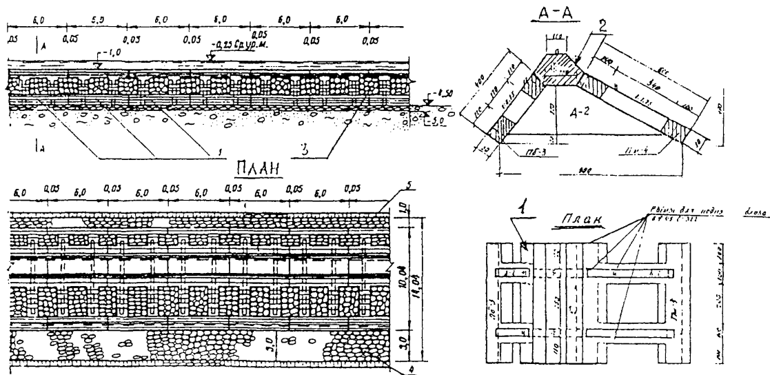
Рисунок 7.26 - Волнолом из шатровых блоков: 1 - шатровый блок; 2 - вкладыш; 3 - бутовый камень; 4 - рисберма перед носком волнолома; 5 - рисберма за задней гранью волнолома
