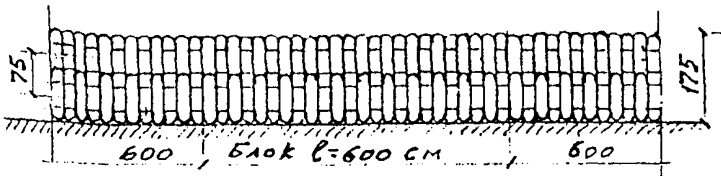
Берма по варианту 2.
