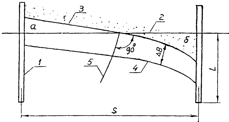
Рисунок 7.14 - Схема переформирования песчаного пляжа в промежутках между бунными сооружениями:
