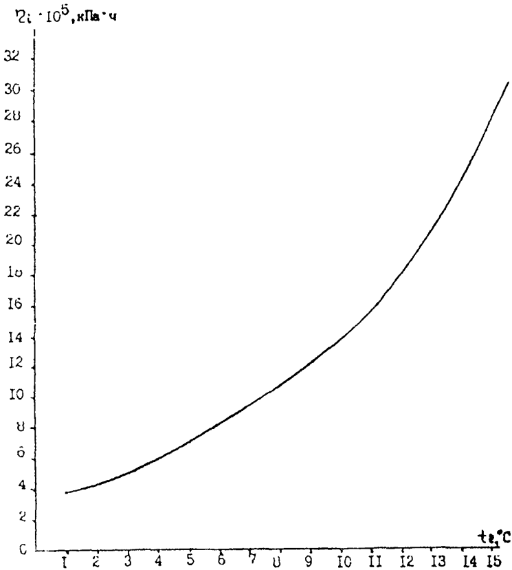
Рисунок 6.6 - Зависимость коэффициента вязкости льда ( \eta_i \cdot 10^5 КПа·с) от температуры льда ( t_i , ^{\circ}\text{C} )
