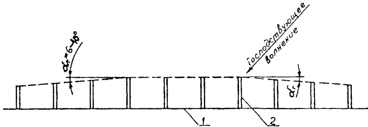
Рисунок 7.16 - Схема уменьшения длины бун на концевых участках системы в условиях песчаных пляжей: 1 - берег; 2 - буна; \alpha_t - угол отклонения линии головных частей бун
