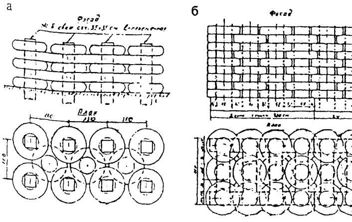
Варианты поперечного сечения бермы
