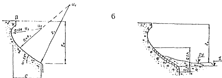
Рисунок 7.11 - Волнозащитная стена с волноотбойным устройством: а - очертание передней грани стены; б - облицовка передней грани стены; л - средний уровень моря
