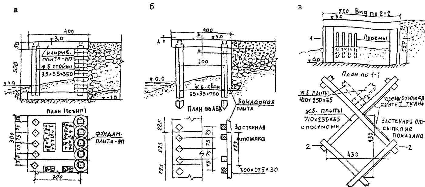
Рисунок 7.29 - Варианты волногасящих стен сквозной конструкции с камерой гашения: а) сборной конструкции на скальном основании; б) свайной конструкции на размываемом основании; в) сборной железобетонной конструкции ромбовидной формы в плане
