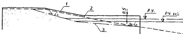
Рисунок 7.15 - Схема профиля буны на берегу с песчаными наносами: 1 - гребень буны; 2 - профиль проектного пляжа с верховой стороны буны; 3 - то же с низовой стороны буны
