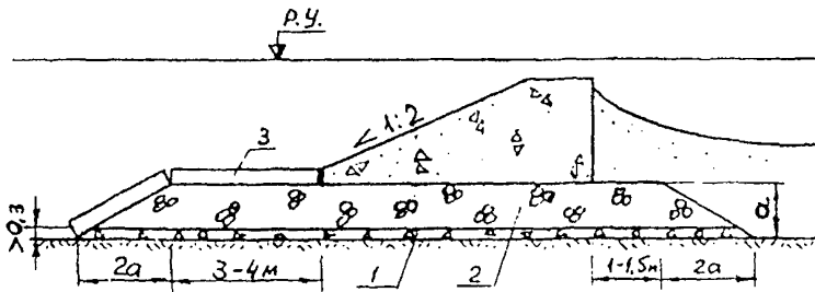
Рисунок 7.25 - Гравитационный подводный волнолом на каменной постели: 1 - щебень; 2 - камень; 3 - берменные плиты
