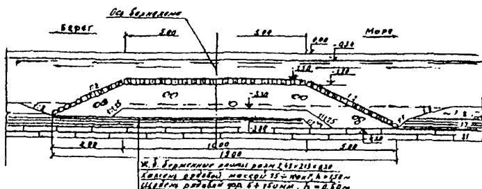
Рисунок 7.27 - Поперечное сечение волнолома распластанный конструкции
