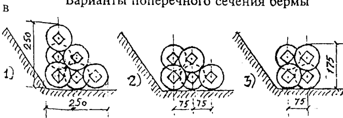
Берма по варианту 2.
