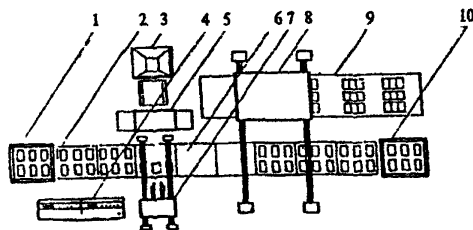
Рис. 2. Система строительства блокированных и индивидуальных жилых домов из мелких бетонных блоков повышенной точности сухого прессования
