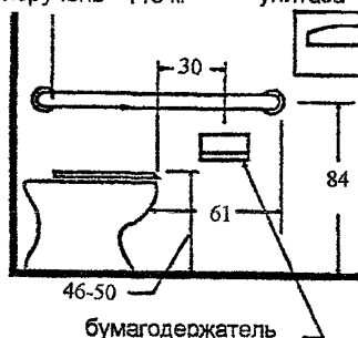
Развертка по боковой стене
