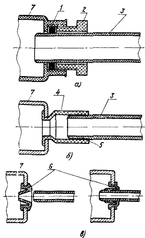
Рис. 9.30 Ввод пластиковых труб в коробки с уплотнением:
