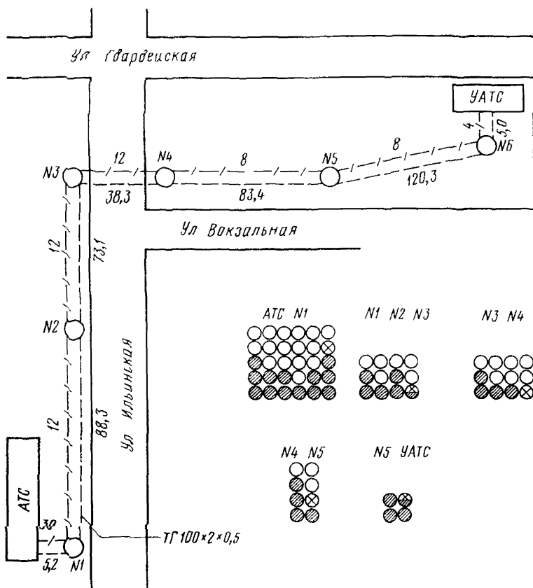
Рис 41 Рабочий чертеж на прокладку кабеля в канализации
