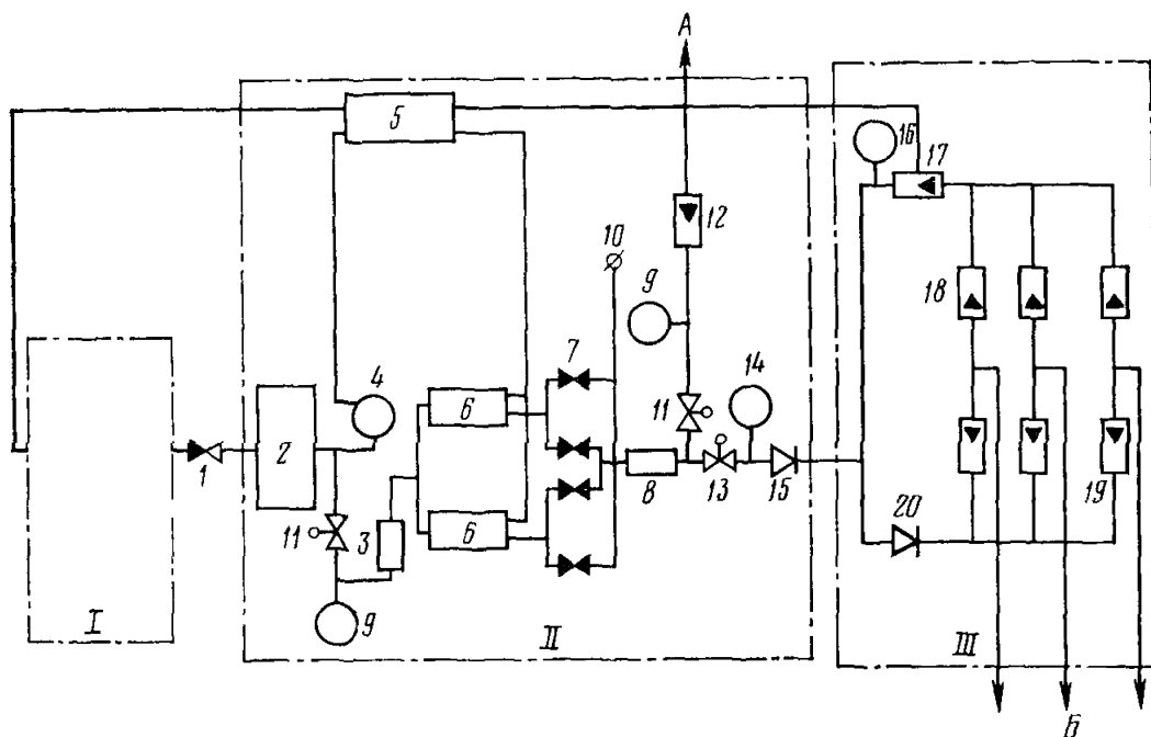
Рис. 122. Функциональная схема КСУ-М:
