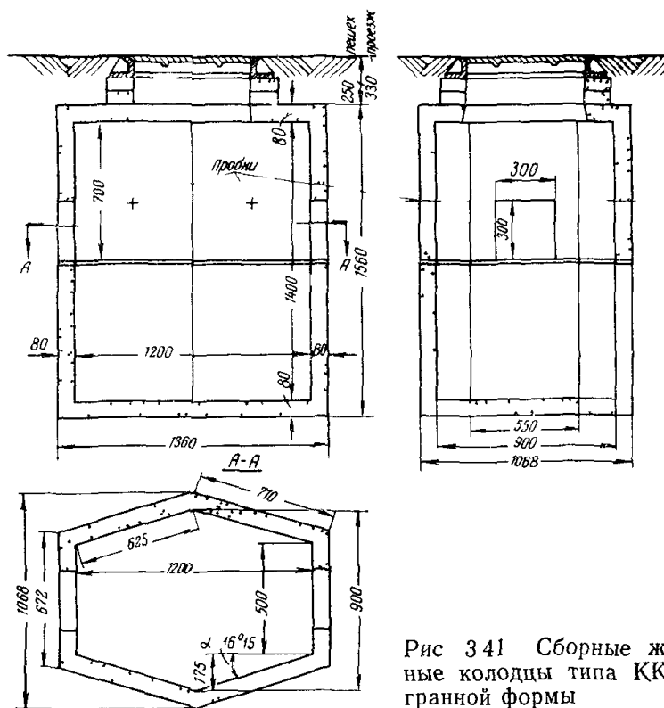
Рис 340 Сборные железобетонные колодцы типа ККС-1
