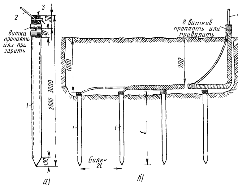
Рис 728 Устройство заземления
