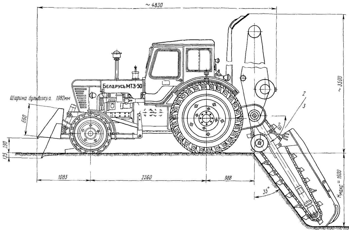
Рис 153 Цепной траншейный экскаватор ЭТЦ-161
