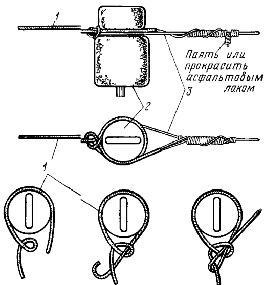
Рис. 737 Соединение изолированного провода типа ПСБАП(В) с голым линейным проводом на пересечениях с электропроводами. 1 — провод ПСБАП(В) 2 — изолятор, 3 — линейный провод
