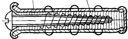
Рис. 9 47. Крепление фасонных скреп шурупами на дюбелях с волокнистым наполнителем
