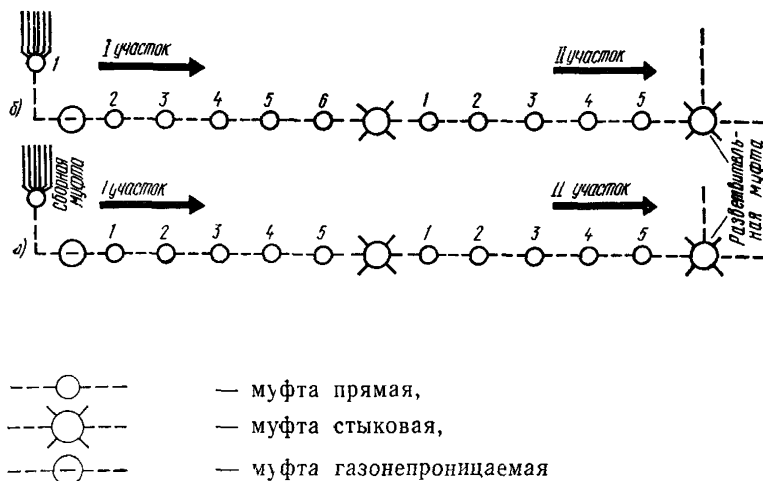
Рис 10.5 Последовательность монтажа муфт кабельных линий ГТС
