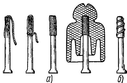
Рис. 7.11. Насадка изоляторов:
