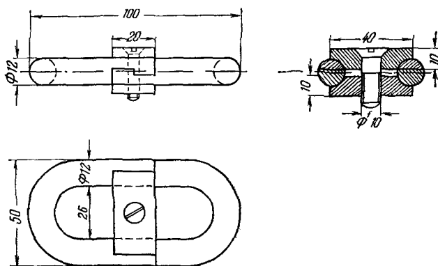
Рис. 4.10. Карабин
