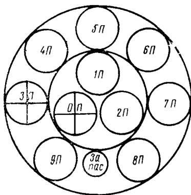
Рис 10 64 Порядок распределения жил по плитам бокса 100х2 в кабеле пучковой скрутки
