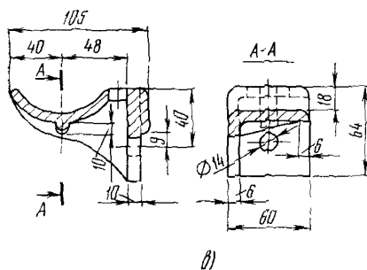
Рис. 362 Консоли кабельные и консольные крючья для смотровых устройств кабельной канализации. а — консоль кабельная чугунная трехместная; б — то же, двухместная; в — то же, одноместная; г — крюк консольный
