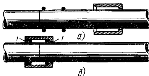
Рис. 3.18. Способ с применением специальных асбестоцементных муфт и резиновых колец: а — наведение специальной асбестоцементной муфты и резиновых колец; б — готовый стык:
