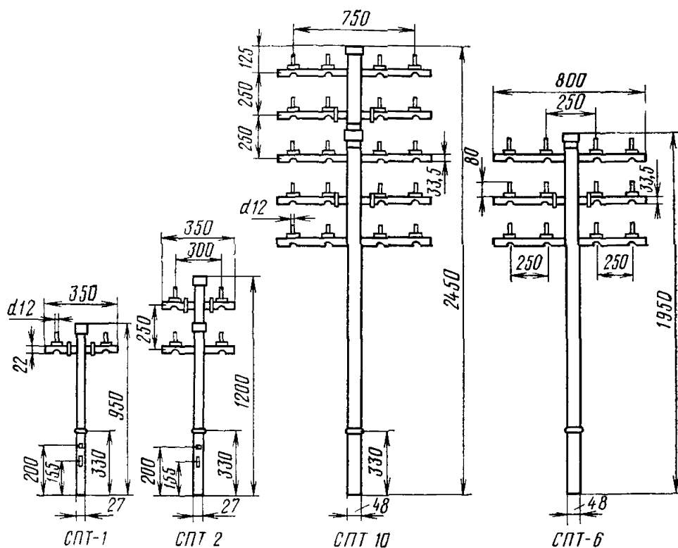
Рис. 8.1. Стоечные опоры
