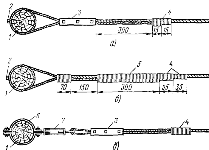
Рис. 7.38. Оконечная заделка стального каната:
