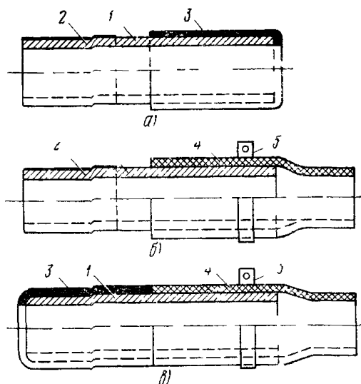
Рис. 10 39. Конструкции переходных манжет:
