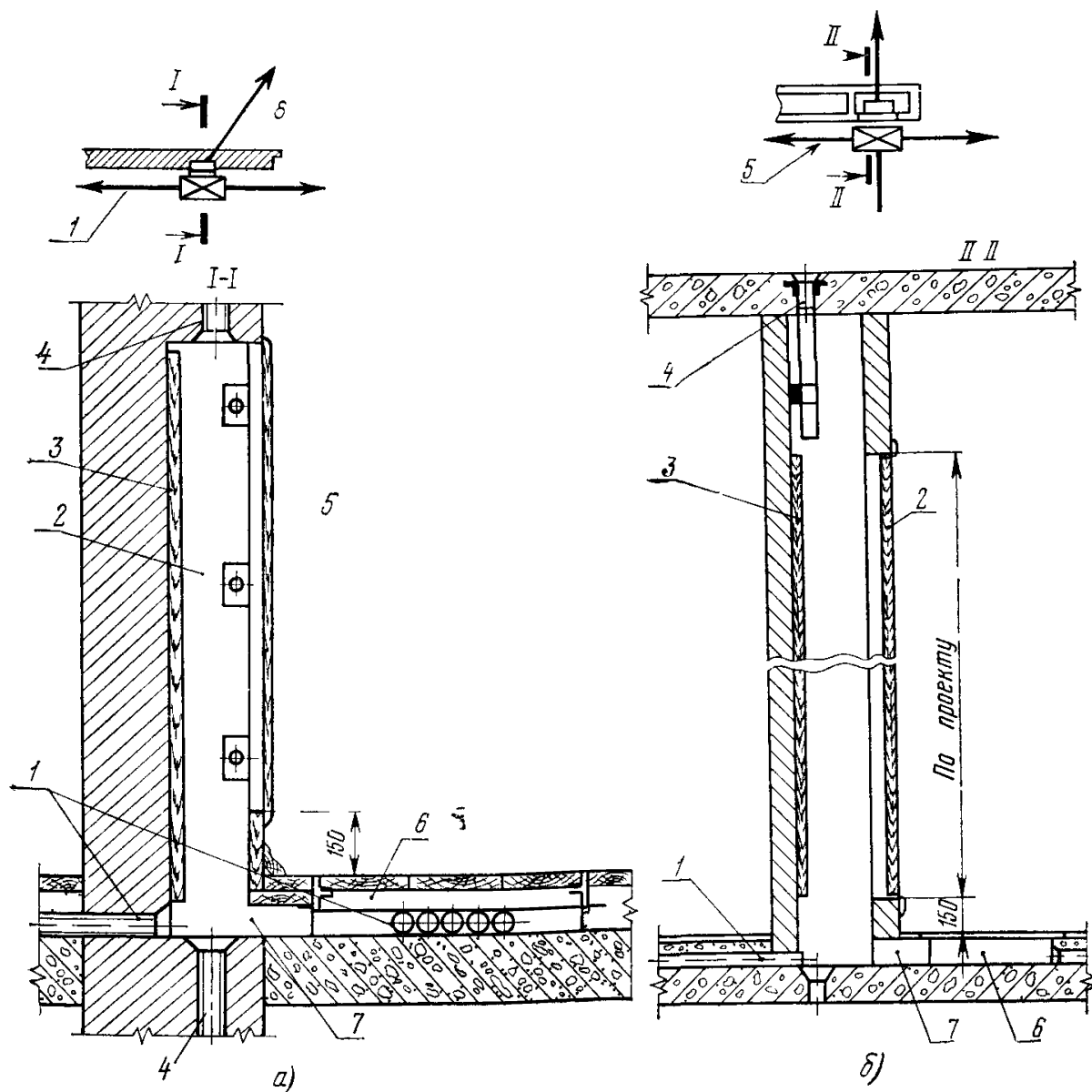
Рис. 9 36 Узел вертикального стояка: а — в капитальной стене; б — в шахте здания:
