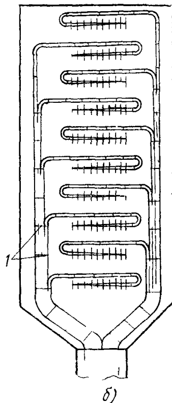
Рис 10 66 Способы вязки пучков жил в боксах а — вязка индивидуальными десятипарными пучками от корешка до плинтов, б — вязка общими жгутами от корешка до ответвлений к плинтам 1 — общая вязка жгутов 2 — индивидуальная вязка каждого десятипарного пучка
