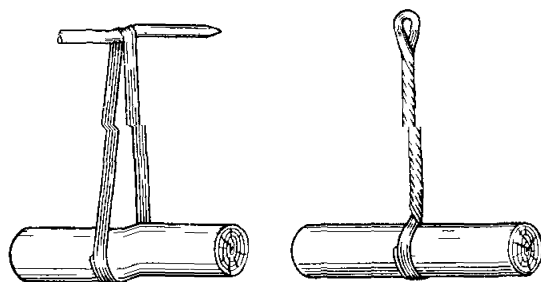
Рис. 7 22. Заделка якорного жгута
