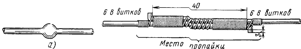
Рис. 736 Сращивание стальных проводов диаметром 3 мм.
