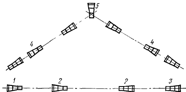
Рис. 7.13. Расположение ям для опор воздушных линий:
