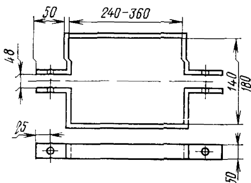
Рис. 7 19 Двухшковый хомут
