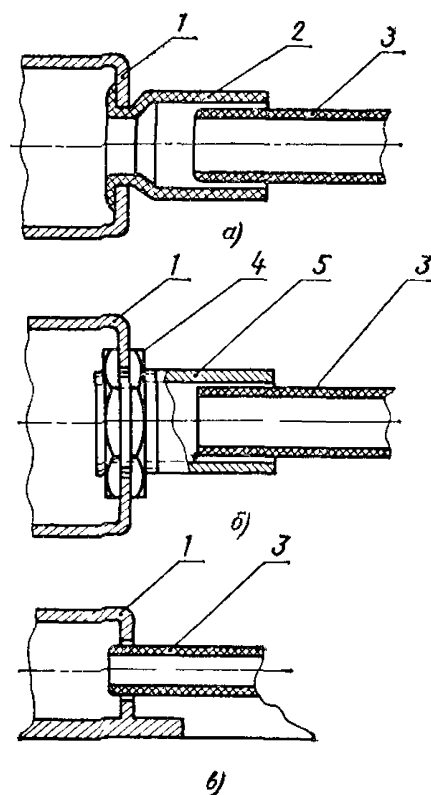
Рис. 9.31. Ввод пластиковых труб в коробки без уплотне- ния:
