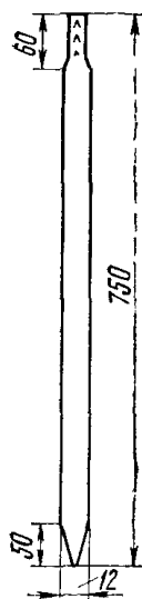
Рис. 8.2. Стальной штырь
