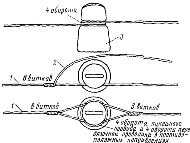
Рис 817 Вязка проводов на изоляторах промежуточной стойки
