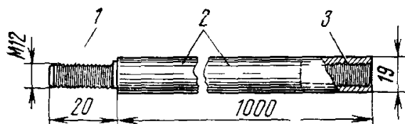
Рис 43 Палка винтовая
