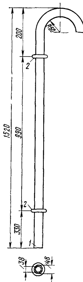
Рис. 8.3. Выводная труба:
