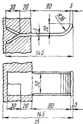
Рис. 362 Консоли кабельные и консольные крючья для смотровых устройств кабельной канализации. а — консоль кабельная чугунная трехместная; б — то же, двухместная; в — то же, одноместная; г — крюк консольный
