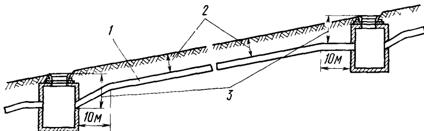
Рис 32 Схема прокладки трубопровода на местности, имеющей естественный уклон
