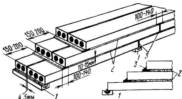
Рис 3.27. Блок из нескольких рядов бетонных труб:
