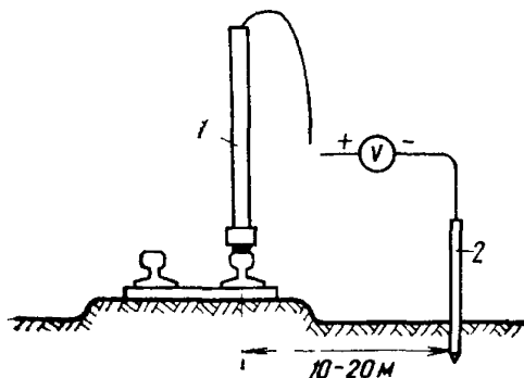
Рис. 14.11. Схема измерения потенциалов рельс электрифицированного транспорта относительно земли: 1 — деревянная штанга со стальным накопечником, 2 — стальной электрод
