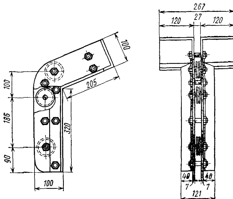
Рис. 4.16. Колено блочное
