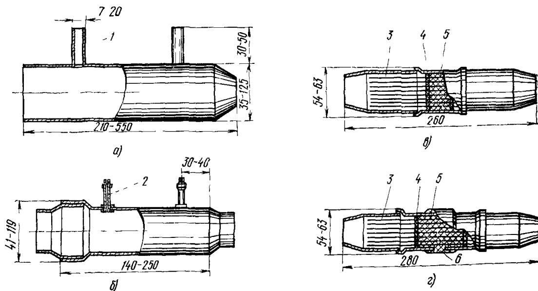
Рис. 12.17. Газонепроницаемые муфты:
