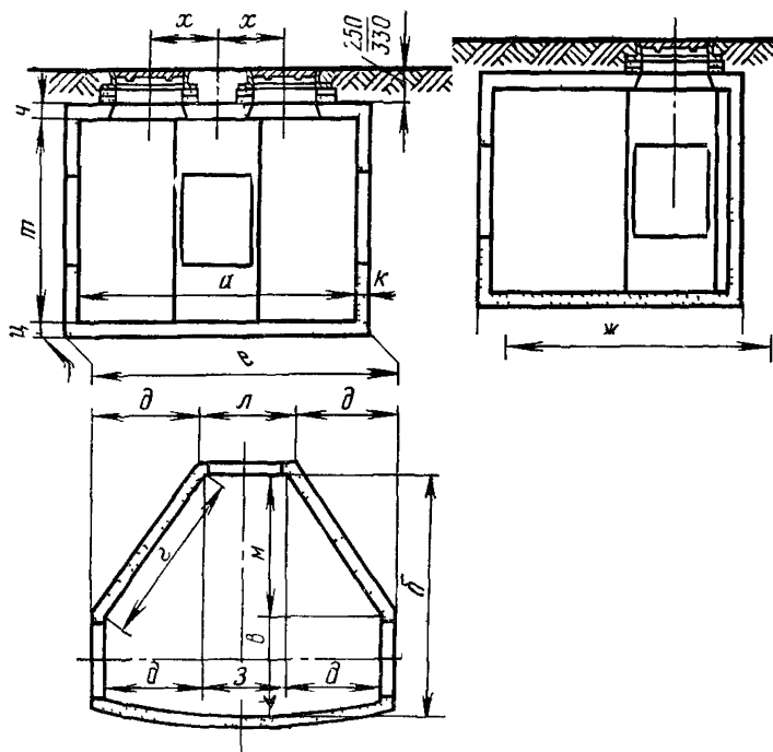
Рис 3 52 Монолитные железобетонные станционные колодцы для станции на 3000, 6000, 10 000 и 20 000 номеров
