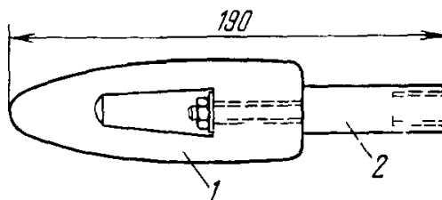
Рис 44 Наконечник для винтовых палок
