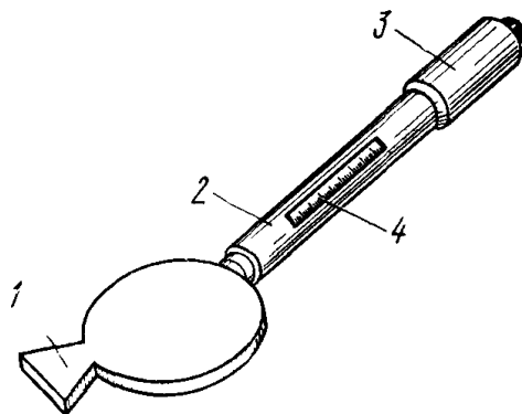
Рис. 330 Нагревательный диск 1 — выступ для нагрева диска пламенем паяльной лампы или газовой горелки, 2 — дюраlevая трубка 3 — деревянная или пластмассовая рукоятка, 4 — электроконтактный термометр или термодатчик
