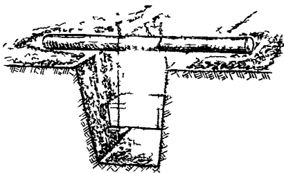
Рис 21 Подвеска подземного сооружения с заключением в короб
