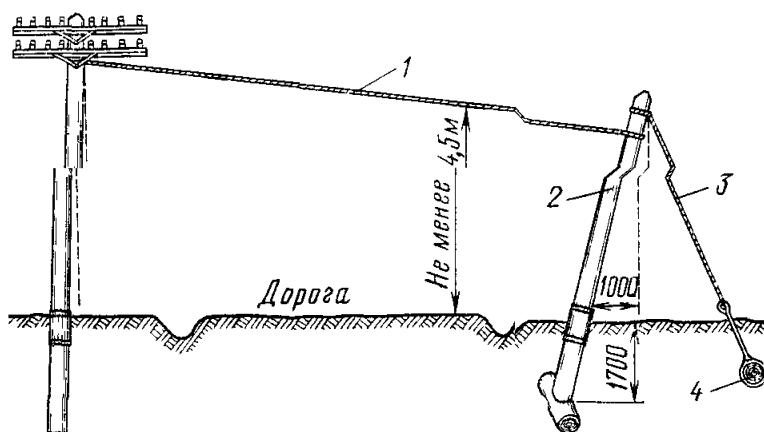
Рис. 7 23 Устройство оттяжного столба.
