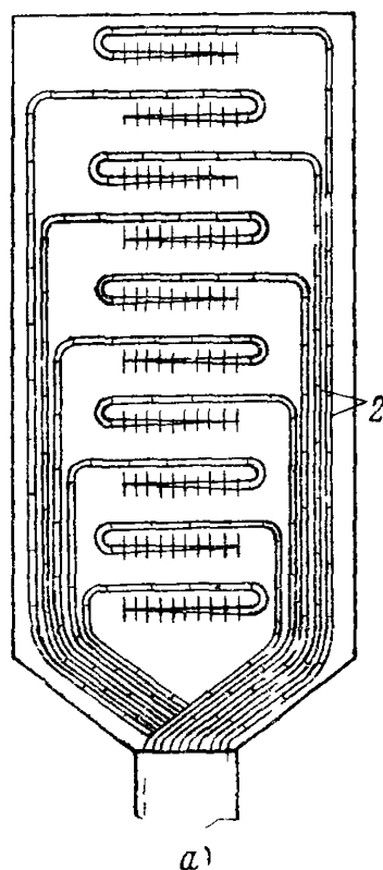
Рис 10 66 Способы вязки пучков жил в боксах а — вязка индивидуальными десятипарными пучками от корешка до плинтов, б — вязка общими жгутами от корешка до ответвлений к плинтам 1 — общая вязка жгутов 2 — индивидуальная вязка каждого десятипарного пучка
