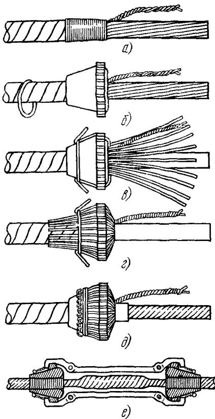
Рис. 10.44. Соединение круглых проволок брони при помощи стяжной муфты с грушевидными вкладышами а — припайка жгута из медных проволок; б — навигание стального кольца и посадка вкладыша; в — фиксация вкладыша двумя проволоками брони; г — укладка всех проволок брони на вкладыше; д — отгибание концами бронепроволок стального кольца и наложение бандаж из линейной проволоки диаметром 3 мм; е — установка корпуса муфты
