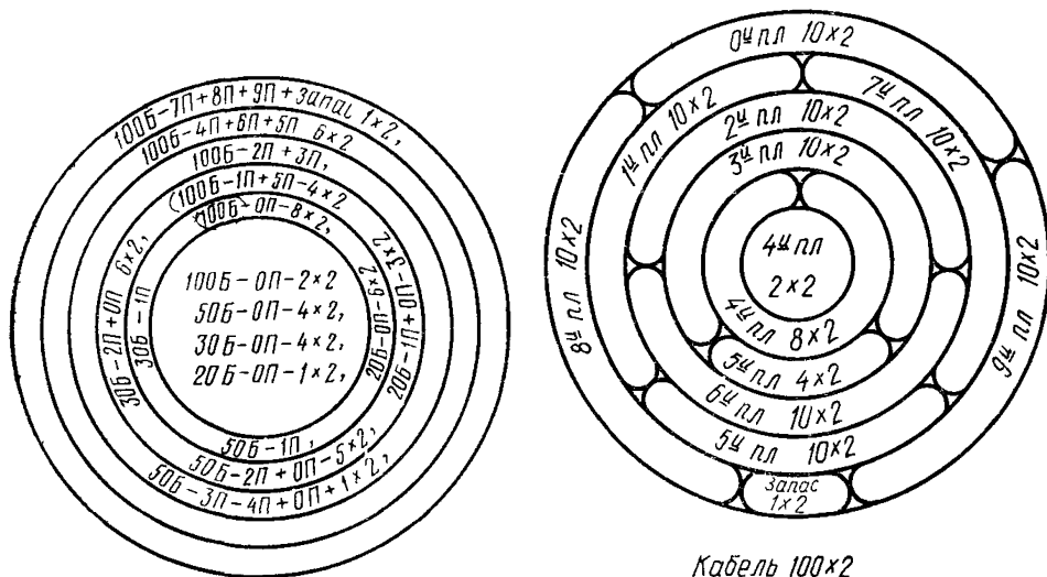
Рис 10 63 Порядок распределения жил по плитам боксов 20х2 30х2, 50х2 и 100х2:
