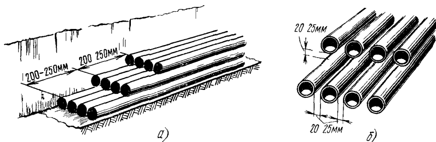
Рис 3 12 Положение труб в блоке
