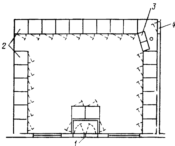
Рис. 13.9. Переговорный павильон таксофонов:
