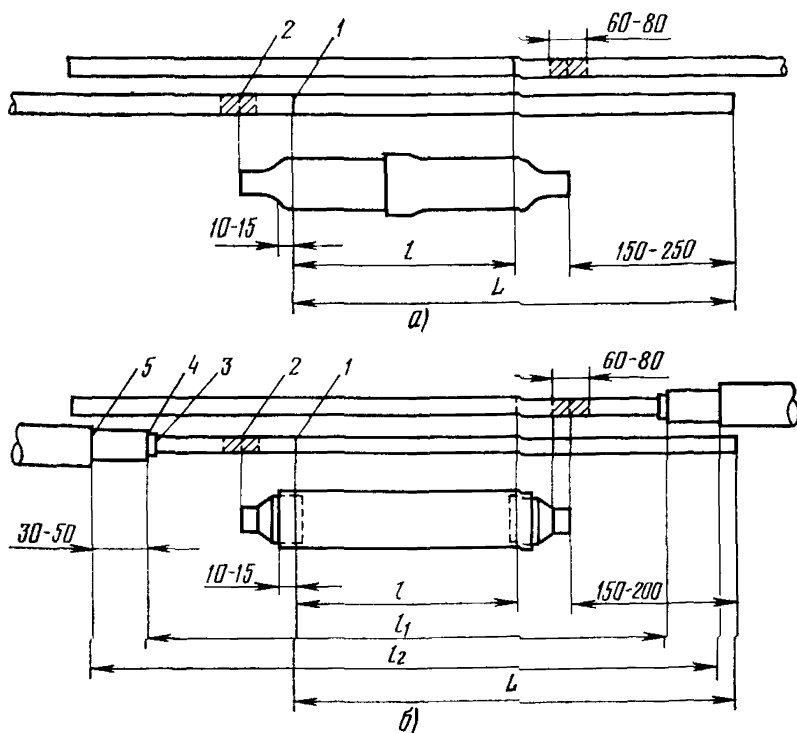
Рис. 108. Размеры разделки кабелей марок ТГ и ТБ:
