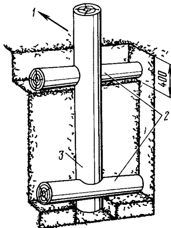
Рис 7118 Укрепление опоры лежнями
