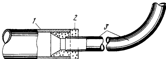
Рис. 9.7. Сопряжение изогнутой стальной трубы с асбестоцементной
