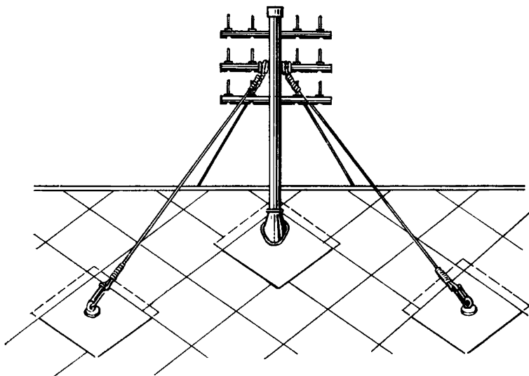
Рис. 8.12. Установка стоечных опор на неметаллических крышах
