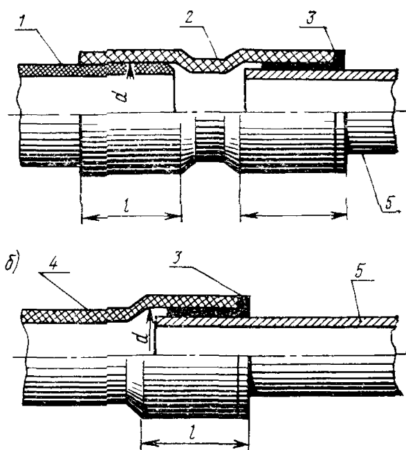
Рис. 9.29. Соединение винипластовых труб со стальными с помощью: а — винипластовой муфты с уплотнителем; б — раструба с уплотнителем: 1 — труба винипластовая, 2 — муфта винипластовая с двумя раструбами, 3 — уплотнитель резиновый, 4 — труба винипластовая с раструбом; 5 — труба стальная
