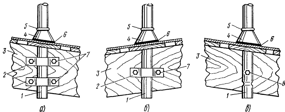
Рис. 8.5. Крепление стоек:
