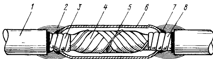
Рис. 10 38. Восстановление стальной гофрированной оболочки свинцовой муфтой:
