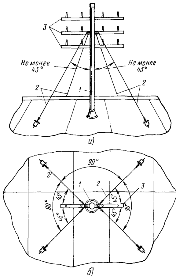
Рис. 8.8. Расположение оттяжек стойки:
