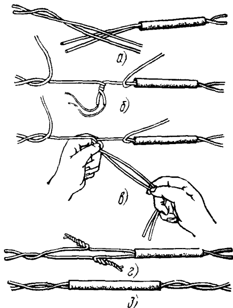
Рис. 10.18. Процесс пожильного сращивания жил ручной скруткой с изолированием пар общей гильзой:
