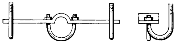
Рис. 8.18. Отходная планка
