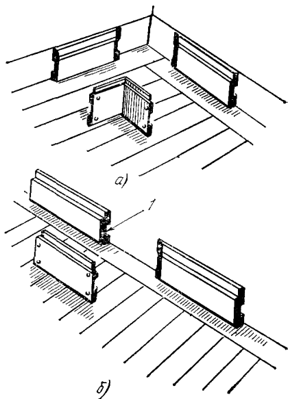
Рис. 9.16. Плинтус с каналом скрытой проводки:
