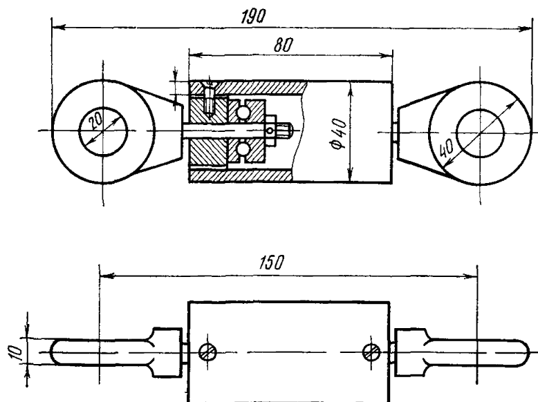
Рис 4 13 Компенсатор кручения
