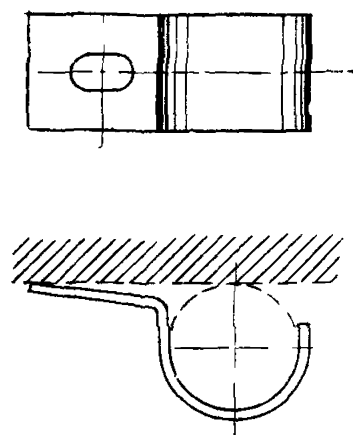
Рис 9 43 Скрепа (скоба) фигурная (фасонная)
