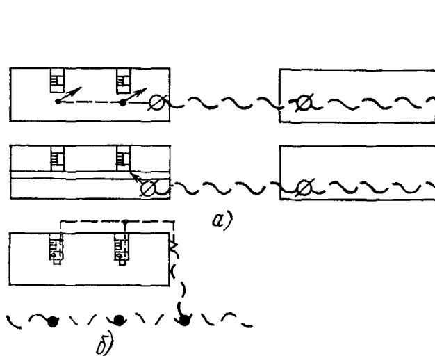
Рис 910 Варианты устройства воздушных вводов в здания
