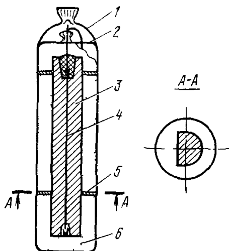
Рис 14 26 Протектор ПМ 10 У/2 МЛ16 в заводской упаковке
