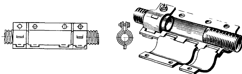
Рис. 9.33 Муфты-коробки типа КБ
