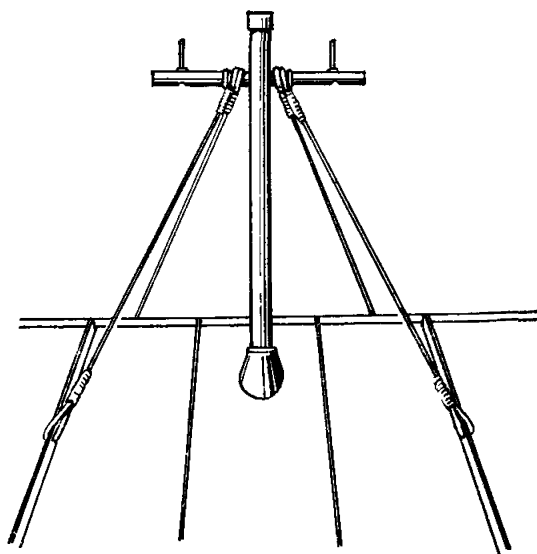
Рис. 8.9. Установка стойки типа СПТ-1
