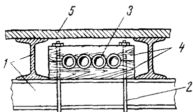
Рис 3 36 Прокладка трубопровода по мосту на деревянных колодках
