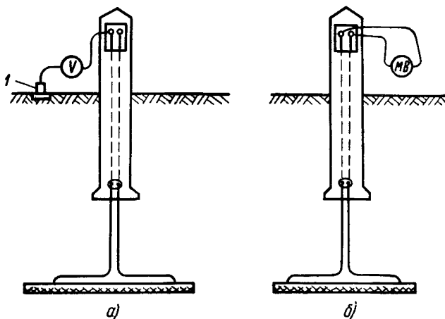
Рис. 14.12. Схема измерения в КИП:
