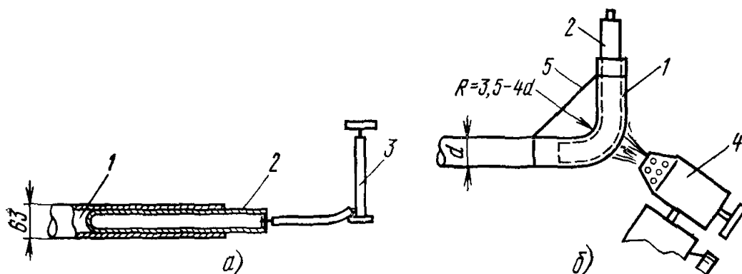
Рис 333 Изгибание полиэтиленовой трубы диаметром 63 мм для вывода на стены зданий а — раздув резинового шланга, б — разогрев изгибаемой трубы.
