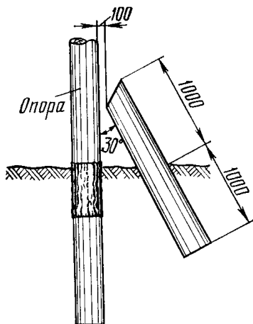
Рис 7.25. Установка отбойной тумбы
