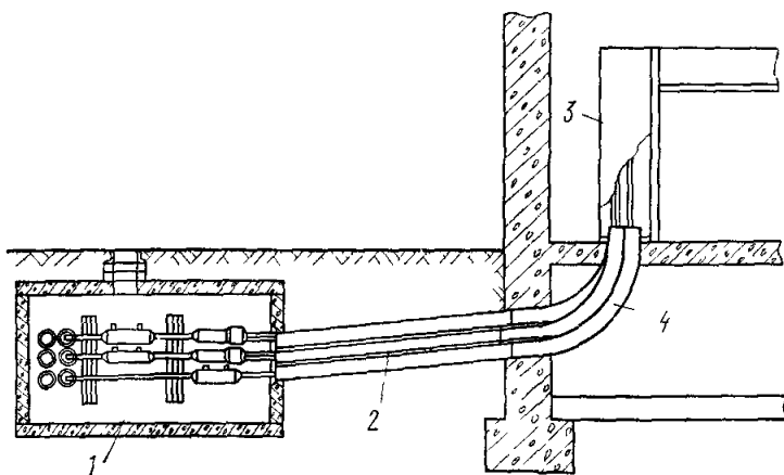
Рис. 373. Ввод кабелей с распайкой в станционном колодце:
