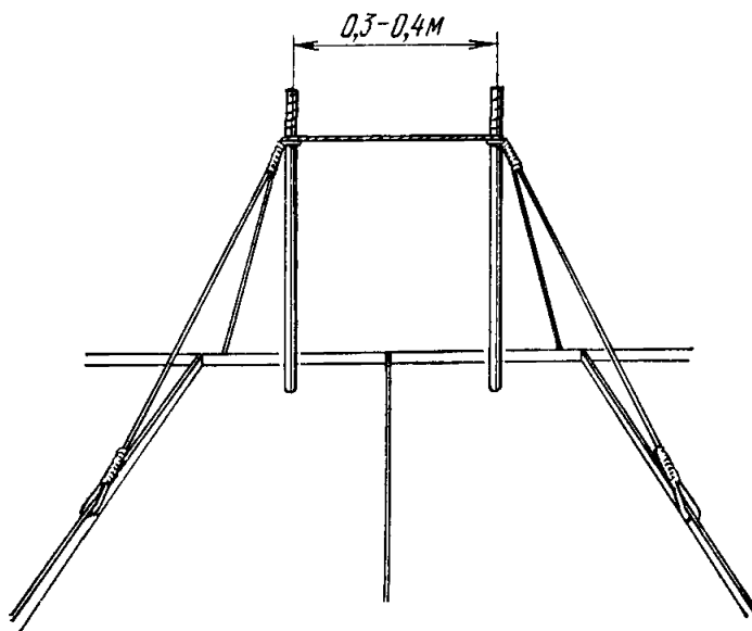
Рис. 8.10. Установка пары штырей
