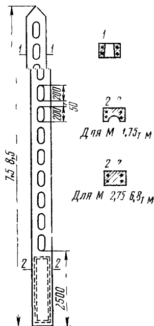
Рис 71 Железобетонная опора
