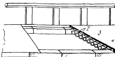
Рис 3 36 Прокладка трубопровода по мосту на деревянных колодках
