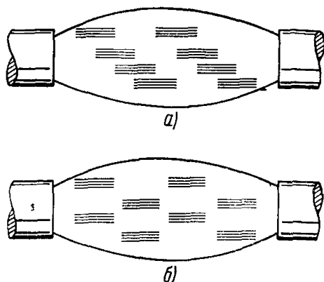
Рис. 10.21. Размещение скруток жил по длине муфты:
