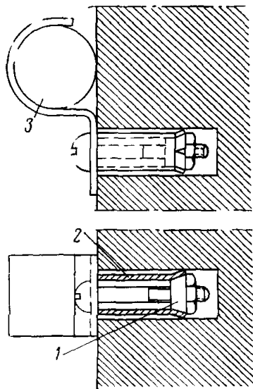
Рис 9 46 Крепление фасонных скреп винтами с распорными гайками:
