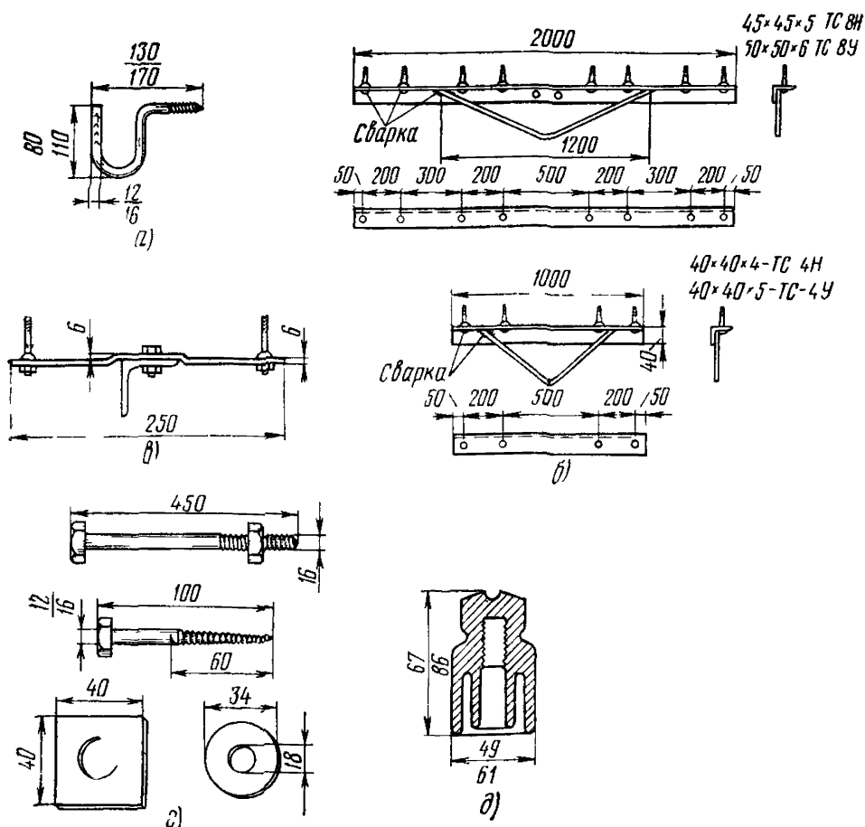
Рис. 7.4 Арматура столбовых линий а — крюки типов КН-12 и КН-16; б — стальные траверсы восьми- и четырехштырные с приваренными штырями и подкосами; в — отходная планка, г — болт, шуруп с шестигранной головкой и шайбы; д — изоляторы типов ТФ-12 и ТФ-16
