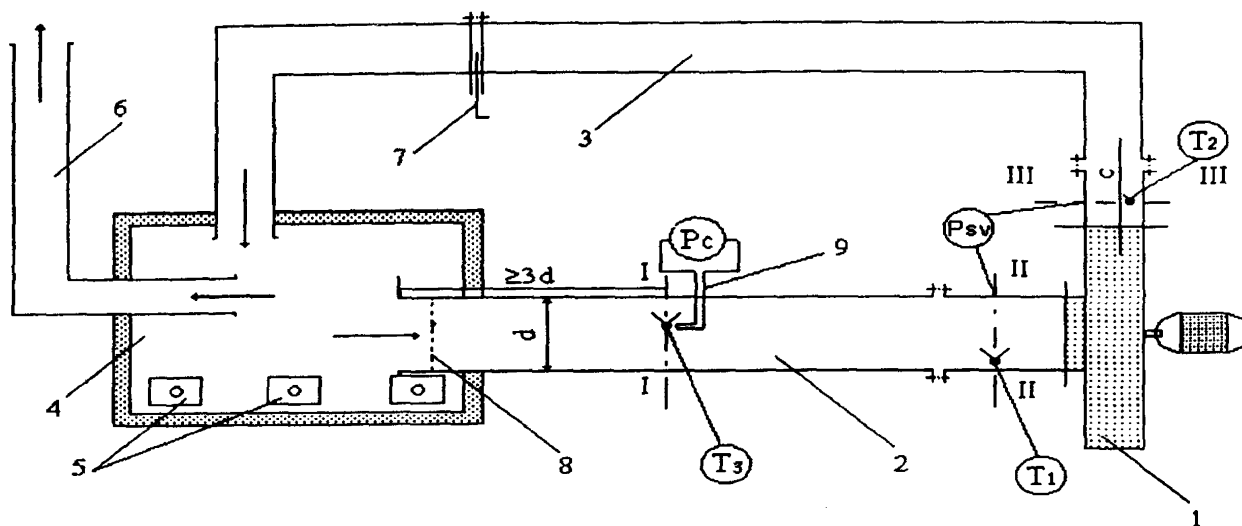
Рис. 1.1. Схема стенда для испытания вентиляторов:
