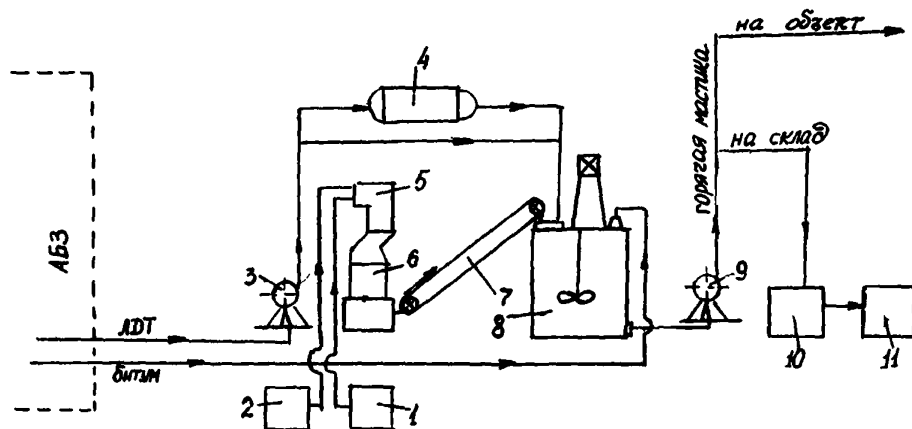
Рис.1. Технологическая схема приготовления полимерно-битумной мастики на АБЗ I - склад для АДТ; 2 - склад для асбеста; 3,9-насосы; 4 - теплообменник; 5 - пневматический нож (дробилка); 6 - сушилка; 7 - транспортер; 8 - котел-смеситель; 10 - брикетные формы; 11 - склад для хранения готовой мастики
