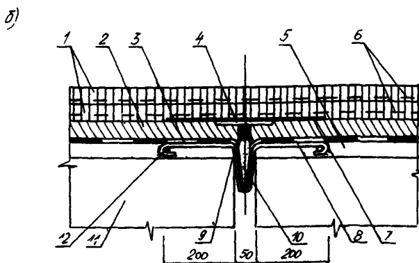
Рис.1. Конструкции деформационных швов закрытого типа: а - с непрерывным асфальтобетонным покрытием; б - с армированным покрытием; 1-асфальтобетонное покрытие; 2-защитный слой; 3-гидроизоляция; 4-металлическая пластина, перекрывающая зазор ( \delta = 6-10 встроена в защитный слой); 5-выравнивающий слой; 6-армирующие сетки; 7-отделяющая прокладка; 8-компенсатор; 9-битумная мастика; 10-пористый заполнитель; 11-балка; 12-якорный стержень; 13-уплотнитель
