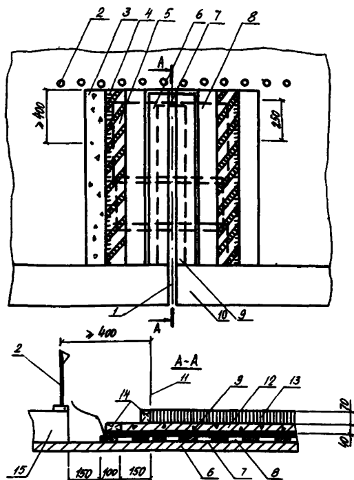
Рис. II. Схема вырубki слоев дорожнoй одежды и их восстановления при реконструкции швов закрытого типа
