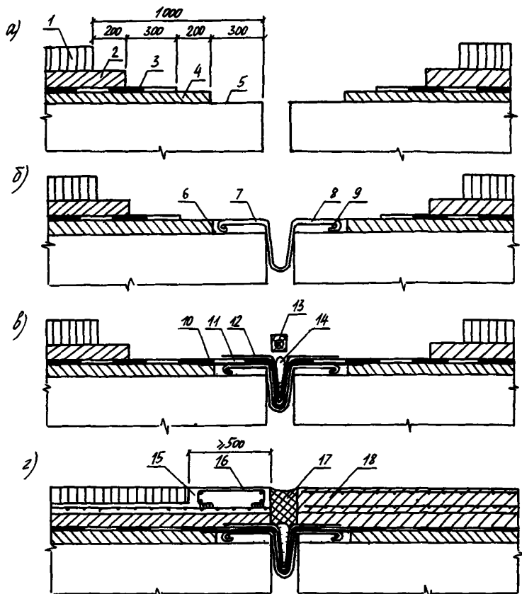
Рис.13. Реконструкция швов заполненного типа:
