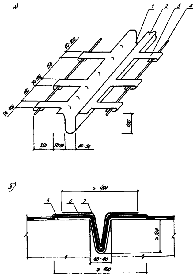
Рис.3. Металлический (а) и неметаллический (б) компенсаторы деформационных швов:
