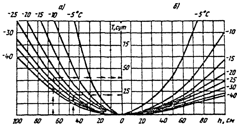
Рис.22. Номограмма для определения времени промерзания T расчищенного от снега ледяного покрова на реках с быстрым (а) и медленным (б) течением при средних (за период промерзания) температурах воздуха (цифры на кривых)
