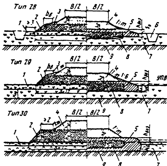
Рис.17. Поперечные профили насыпей на промороженных торфяных основаниях (левая часть – состоящие конструкции в период строительства, правая – в процессе эксплуатации на конец теплых периодов): 1–промороженный слой торфяной залежи; 2–намороженная торфяная плита; 3–боковые призмы из торфа; 4–насыпь из минерального грунта; 5–талые слои торфяной плиты; 6–боковой резерв; 7–талый слой торфяной залежи; 8–мерзлые слои торфяной плиты; 9–минеральное дно болота
