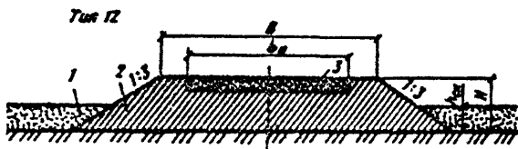
Рис. 6. Поперечный профиль автозимника в насыпи из снега: 1-снежный покров толщиной h_{cm} ; 2-насыпь из уплотненного снега; 3-оледененный слой снега на проезжей части; Н - высота насыпи
