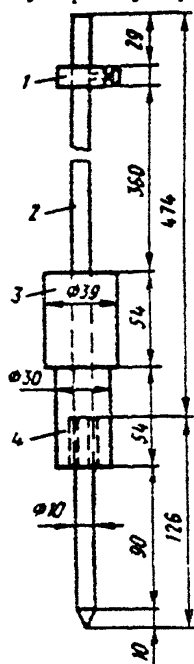
Рис.20. Ударник-зонд Союздорнии: 1—фиксирующая шайба; 2—стальной стержень; 3—гира; 4—упорная шайба
