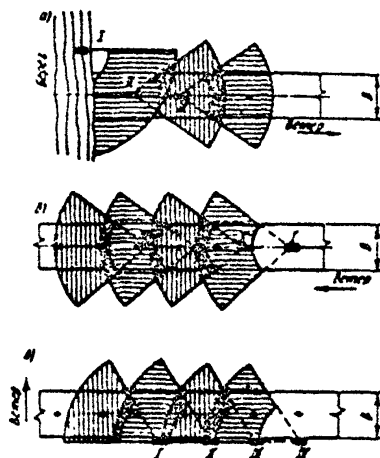
Рис.19. Намораживание ле - довых переправ методом дождевания: а-с берега ; б-при движении агрегата по оси переправы; в-то же, вдоль переправы; • - конт - рольные вехи; -стоянки агрегата; -секторы дождевания; -перекрывае мые зоны; 1-10-последователь - ные стоянки (позиции) агре - гата
