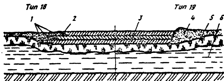
Рис.11. Усиление ледяного покрова методом послойного намораживания льда: 1-пригнанный снег; 2-жерди; 3-намораживаемые слои; 4-вал из снега; 5-естественный ледяной покров; 6-вода
