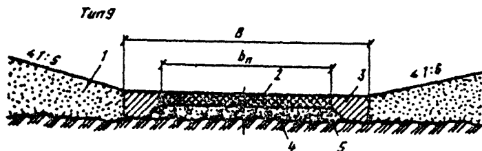
Рис.4. Поперечный профиль автозимника на марях и бугристых вечномерзлых торфяниках: 1—снежный покров; 2—уплотненный или оледеневший снег на проезжей части; 3—уплотненный снег на обочинах; 4—выравнивающий слой из гравия или песка; 5—спланированное мерзлое основание
