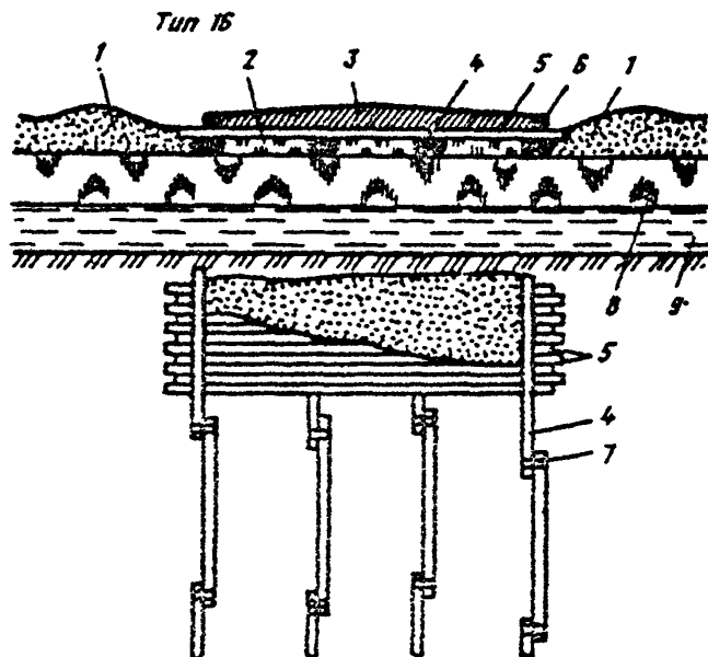
Рис. 9. Конструкция "плавающей" дереволедяной переправы: 1—валик из снега; 2—намороженный слой льда; 3—снежно-ледяное полотно; 4—продольные лежни, a > 20 см; 5—сланевый настил из тонкомерной древесины; 6—колесоотбой, d > 22 см; 7—проволочная скрутка \Phi=8 мм; 8—естественный ледяной покров; 9—вода
