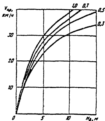
Рис.23. Зависимость критической скорости волны от глубины водоема H при различной толщине льда h_{л} , м (цифры на кривых)
