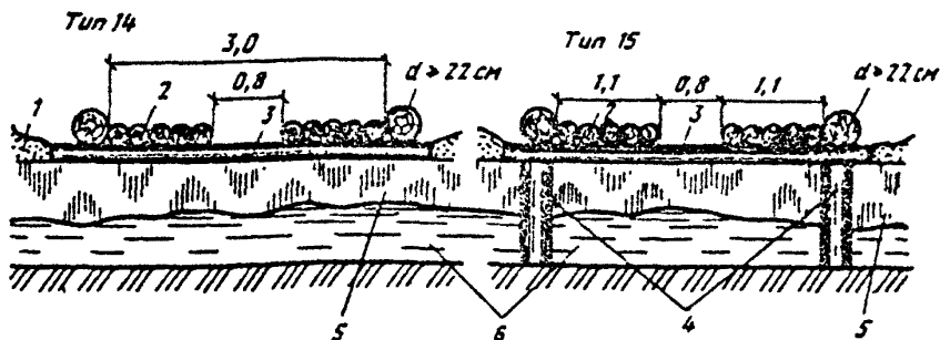
Рис. 8. Усиление ледовых переправ деревянным настилом: 1—снежный покров; 2—колесопроводы, d \geq 22 см; 3—поперечины, d \geq 18 см; 4—стойки, d \geq 20 см; 5—естественный ледяной покров; 6—вода
