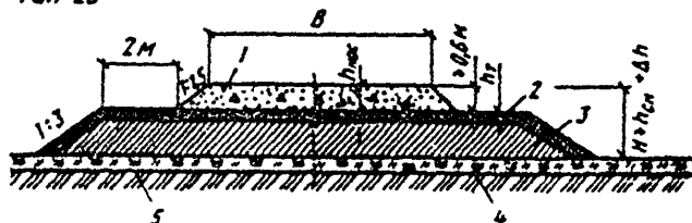
Рис.15. Поперечный профиль автозимника для круглогодичной эксплуатации: 1—земляное полотно из минерального грунта; 2—слой теплоизоляции из торфа, мха, опилок и т.п.; 3—снежно-ледяное ядро; 4—естественный мохорастительный покров; 5—мерзлое грунтовое основание
