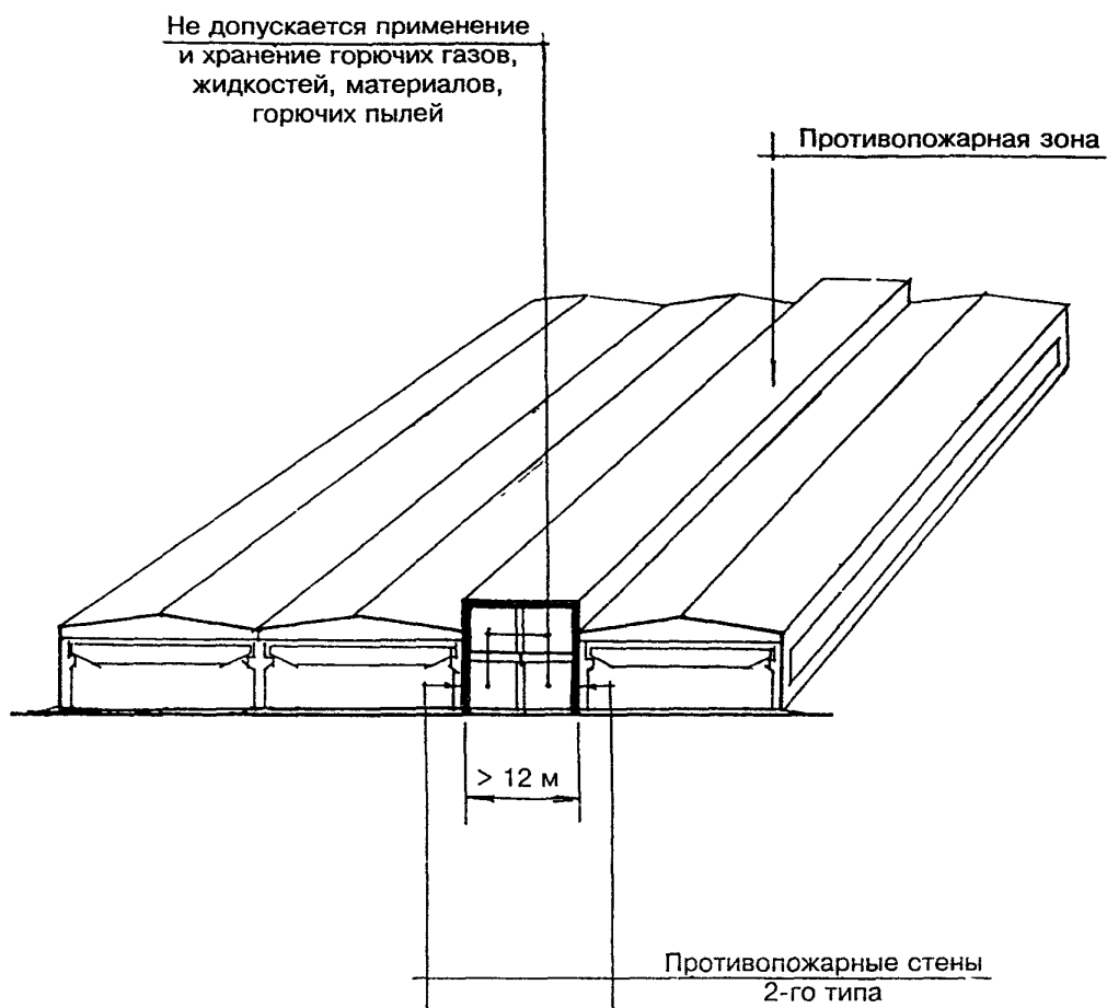
Рис. 9. Противопожарная зона
