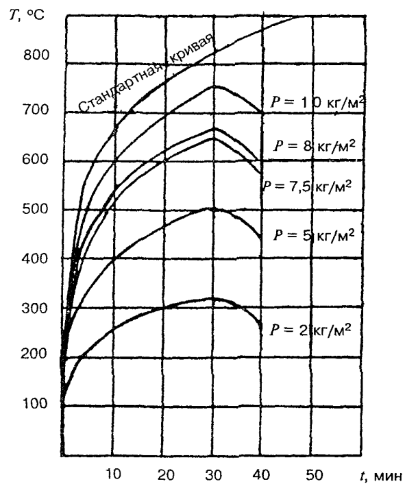
Рис. 4. Температурные режимы ПРН
