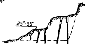
Рис. 5.4. Расположение наклонных скважин на косогорах с уклоном 25—35°
