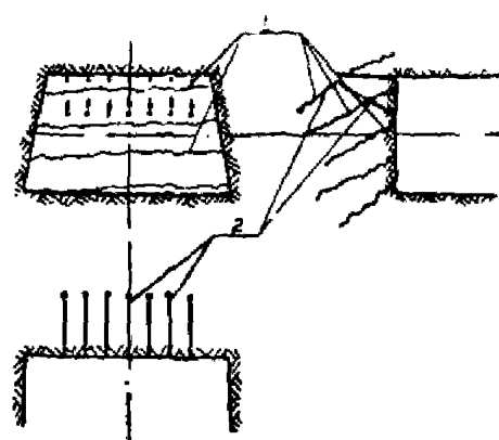
Рис. 2.8. Горизонтальный верхний клиновидный вруб:
