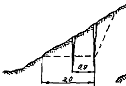
Рис. 5.2. Расположение шпуровых зарядов при проходке троп
