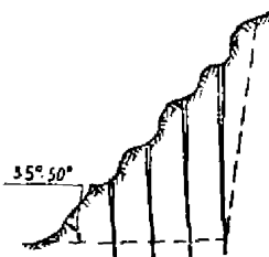
Рис. 5.5. Расположение вертикальных скважин на косогорах с уклоном 35—50°
