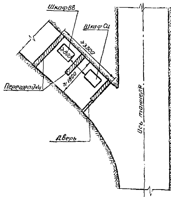
Рис. 7.7. Схема участка хранения в существующей выработке (УПХ до 100 кг ВВ)
