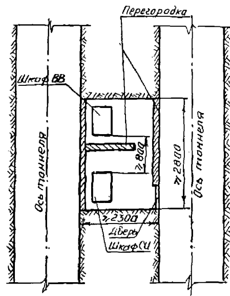
Рис. 7.8. Схема участка хранения в существующей выработке (УПХ до 100 кг ВВ)
