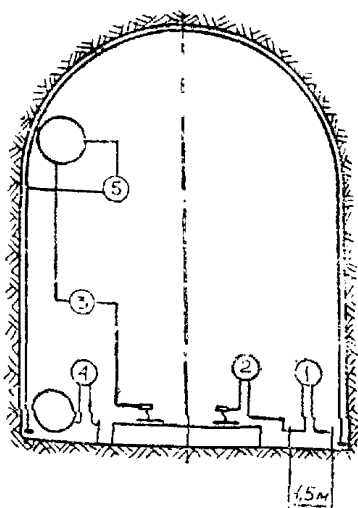
Рис. 8.2. Схема мест измерений блуждающих токов:
