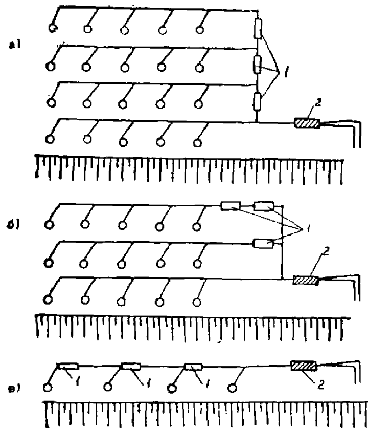
Рис. 4.11. Монтажные схемы короткозамедленного взрывания при помощи пиротехнического реле:
