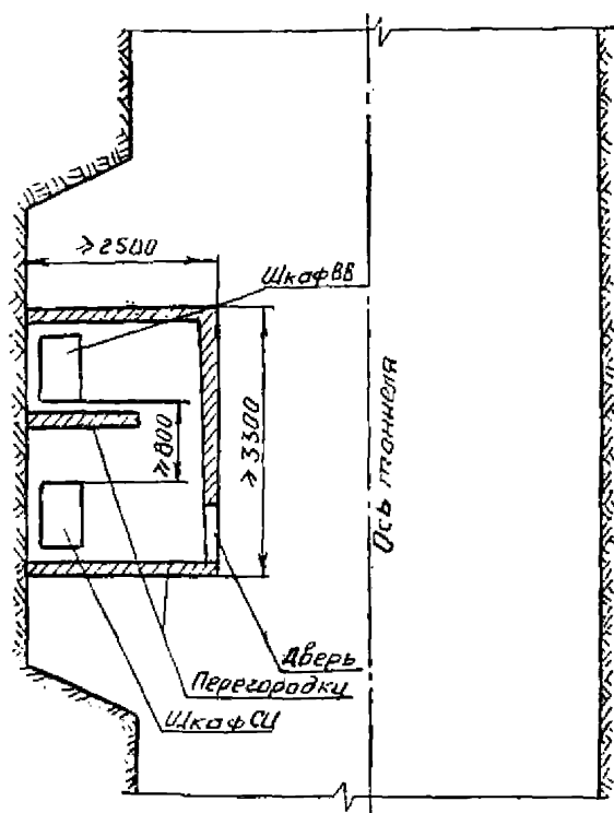
Рис. 7.9. Схема участка пункта хранения (УПХ до 100 кг ВВ)
