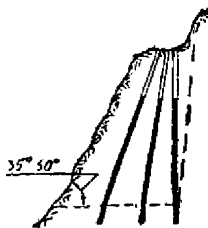
Рис. 5.6. Расположение наклонных скважин на косогорах с уклоном 35—50°
