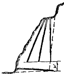
Рис. 5.8. Комбинированное расположение скважин на косогорах с уклоном более 50°
