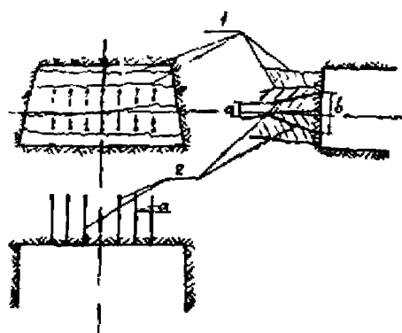
Рис. 2.7. Горизонтальный клиновой вруб:
