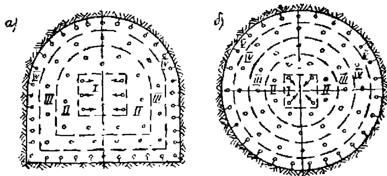
Рис. 4.9. Очередность взрывания шпуров при проходке транспортного тоннеля (а) и ствола (б): а) I—врубовые шпур; II, III—отбойные шпур; IV—контурные шпур; б) I—врубовые шпур; II, III, IV—отбойные шпур; V—контурные шпур
