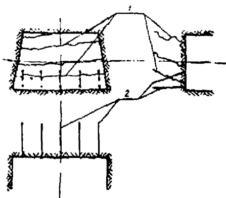
Рис. 2.9. Горизонтальный нижний клиновидный вруб:
