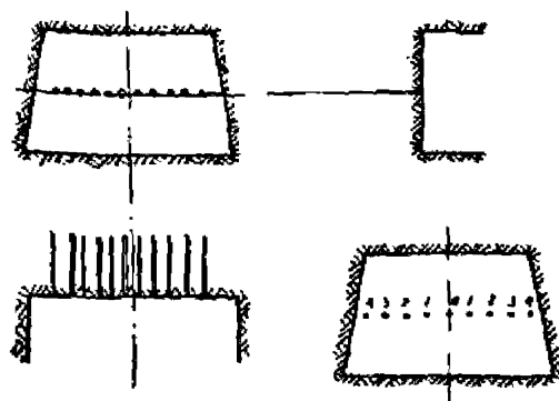
Рис. 2.10. Щелевой (горизонтальный) вруб:
