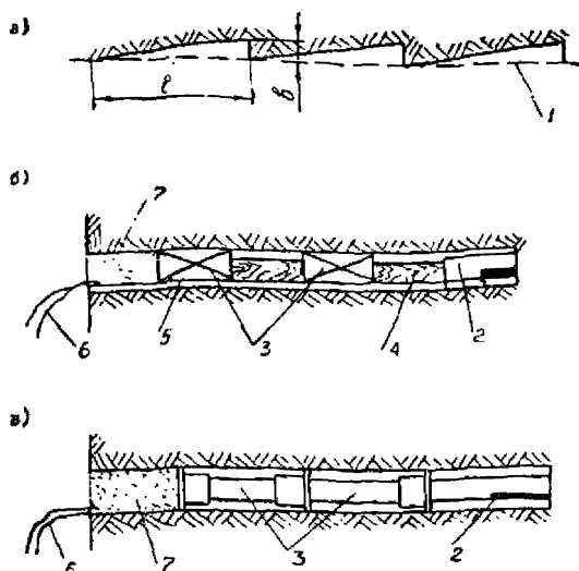
Рис. 2.14. Расположение контурных шпуров и конструкция зарядов для контурных шпуров:
