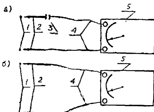
Рис. 8.1. Способы подключения ампервольтметра для измерения напряжений и блуждающих токов: а—при измерении переменных величин; б—при измерении постоянных величин; 1—точка измерения; 2—изолирующий щуп; 3—разделительный конденсатор; 4—соединительный провод; 5—ампервольтметр
