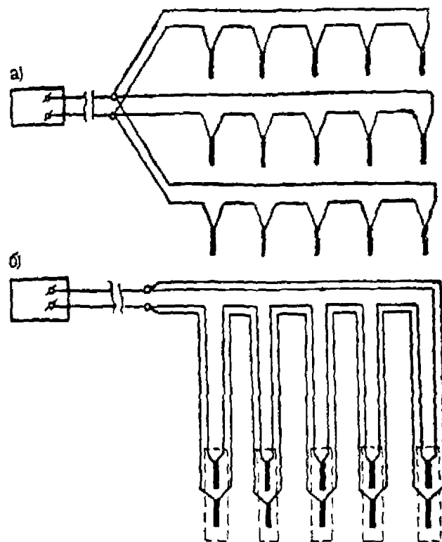
Рис. 4.3. Последовательно-параллельное соединение электродетонаторов:
