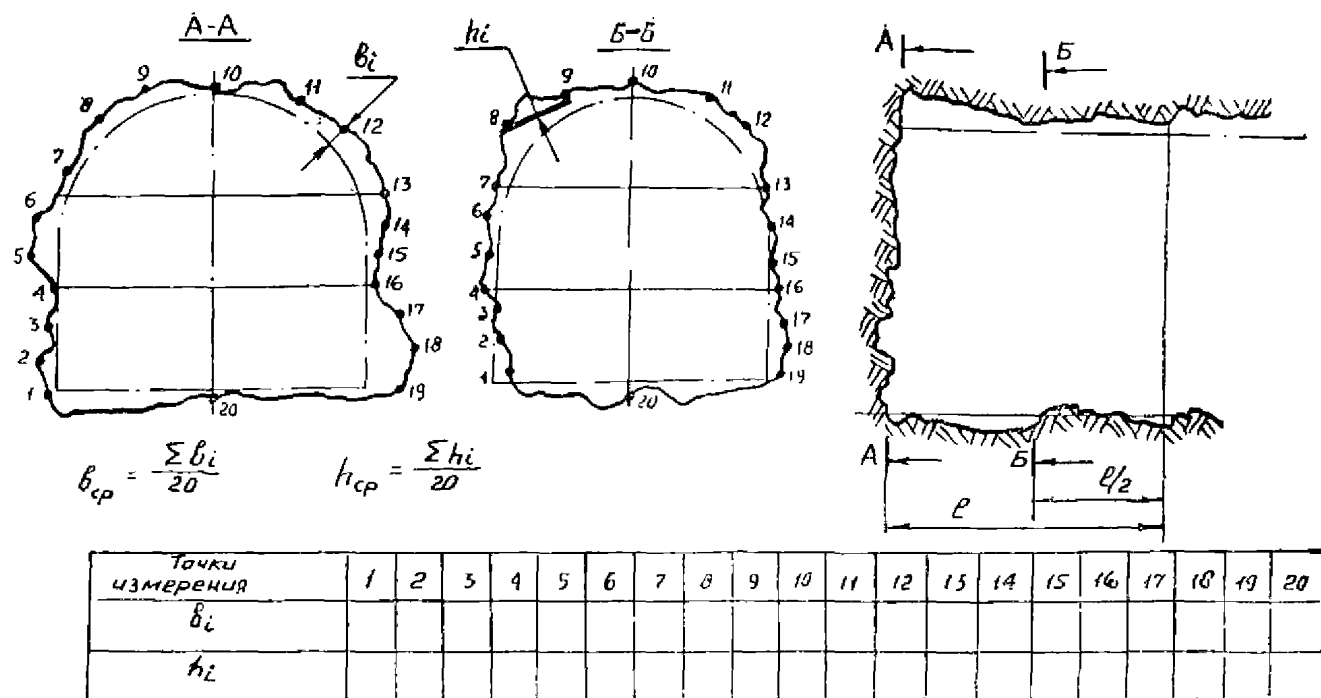
Рис. П.4.1. Схема измерения переборов и параметров состояния поверхности контура
