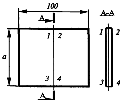
Рис. 1. Вид образца ленты: a - размер, равный ширине ленты. Размеры в мм
