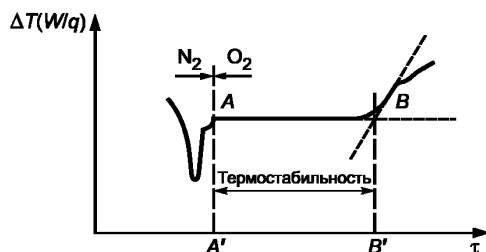
Рисунок 1 — Типичная кривая окислительной термостабильности полиэтилена
