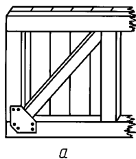
Металлическая скоба
