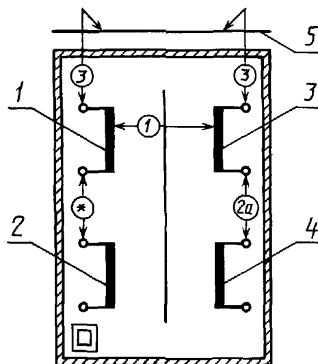
1 — первичная 1; 2 — первичная 2; 3 — вторичная 1; 4 — вторичная 2; 5 — металлическая фольга
