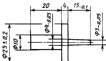
Рисунок 4 — Испытательный стержень
