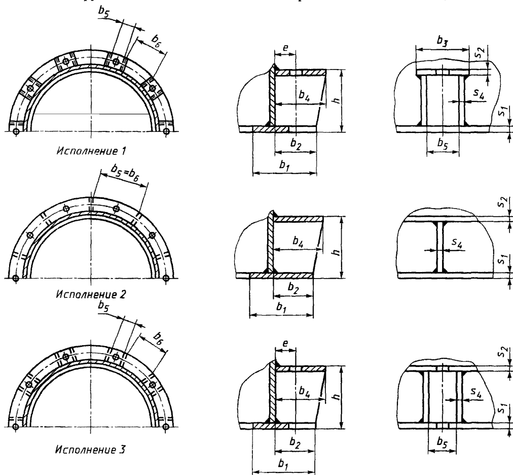
Рисунок 3 — Опорный узел
