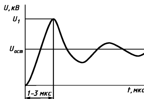
Рисунок Д.2 — Форма грозовых импульсов, характерная для точек присоединения a, в, з, д на рисунке Д.1.
