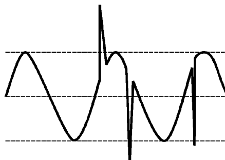
Рисунок А.3 — Импульсы напряжения
