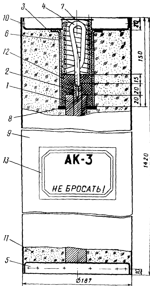
Рис.3. Заземлитель анодный АК-3:
