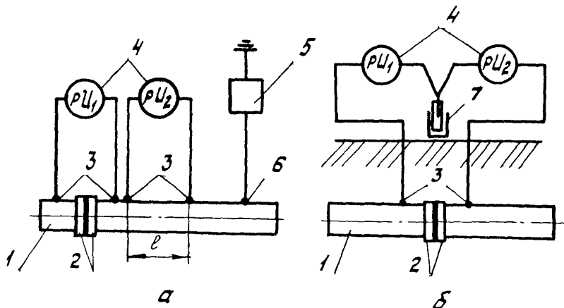
Рис.34. Схемы включения измерительных приборов и устройств при опробовании и наладке изолирующих фланцев трубопровода:
