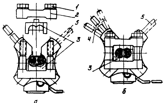
Рис.7. Зажимные узлы приспособления МИ-230А:
