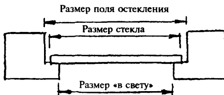
Рисунок А.1 — Определение размеров светопрозрачного заполнения
