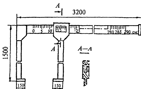
Рисунок 8 — Измерительный шаблон
