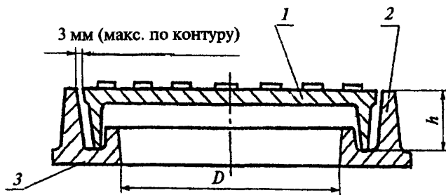
Рисунок А.1 — Люк общего назначения
