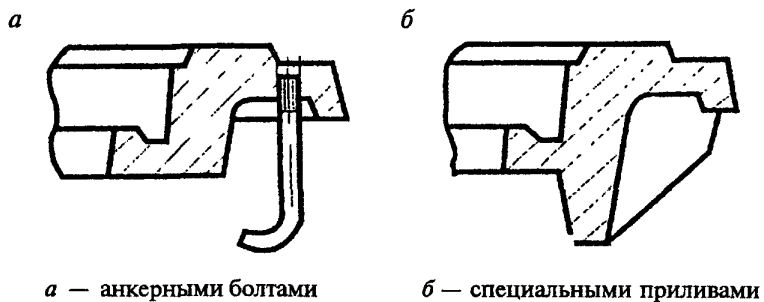
Рисунок А.4 — Усиленная заделка корпуса люка
