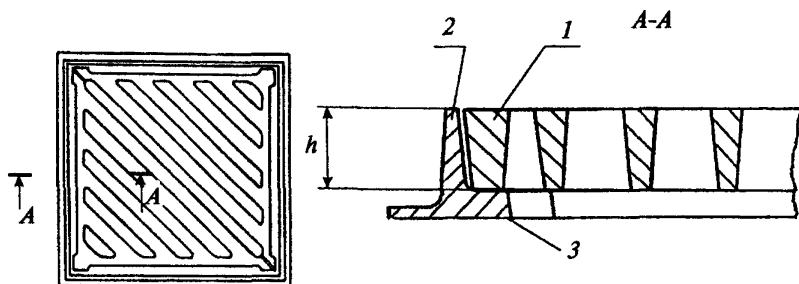
Рисунок Б.1 — Дождеприемник ливнесточного колодца
