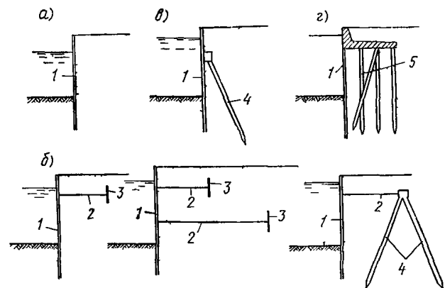
Рис. 2. Основные виды шпунтовых и свайных подпорных стен а — безанкерные, б — заанкеренные одной или двумя тягами к плитам или сваям, в — заанкеренные к наклонным сваям, г — установленные на свайном фундаменте 1 — шпунт 2 — анкерная тяга, 3 — анкерная плита, 4 — анкерные сваи, 5 — свайный фундамент
