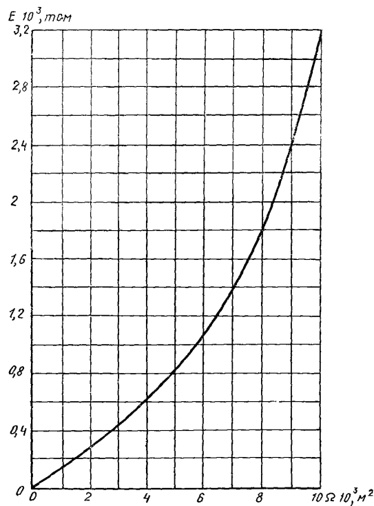
Рис. 7. График для определения энергоемкости предохранительного устройства в зависимости от площади зеркала камер шлюза
