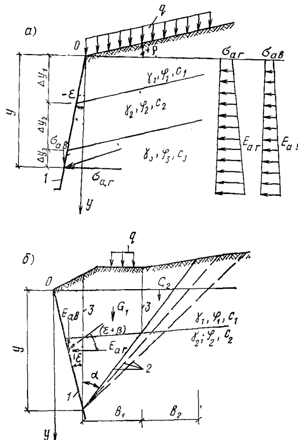
Рис. 1. Схемы к расчету активного давления грунта
