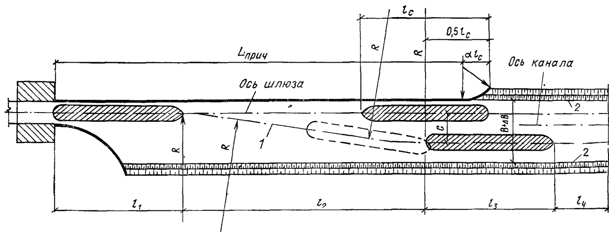
Рис. 9. Схема подходного канала к шлюзу для определения длины причальной линии 1 — траектория движения центра тяжести выходящего из шлюза судна; 2 — граница судового хода
