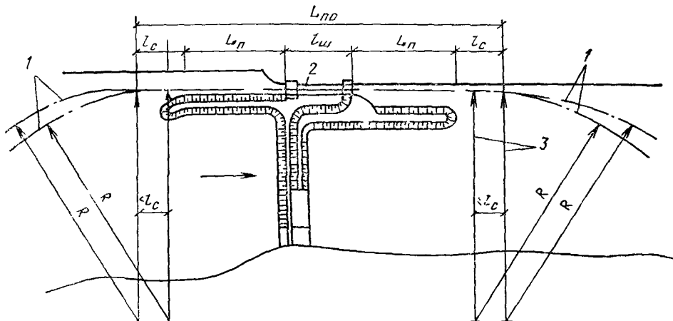
Рис. 4. Схема судоходного шлюза с подходами
