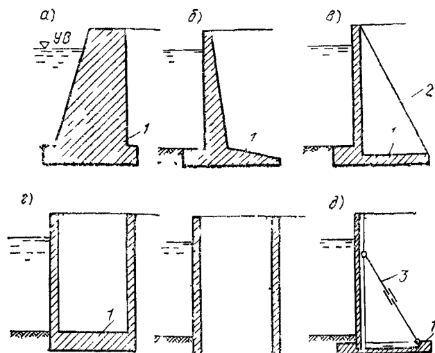
Рис. 1. Основные виды гравитационных подпорных стен а — массивные, б — уголкового, в — контрфорсные, г — ячеистые (с днищем и без днища), д — уголкового сборные с лицевыми элементами, заанкеренными к фундаментным плитам, 1 — фундаментная плита 2 — контрфорс, 3 — анкерная тяга
