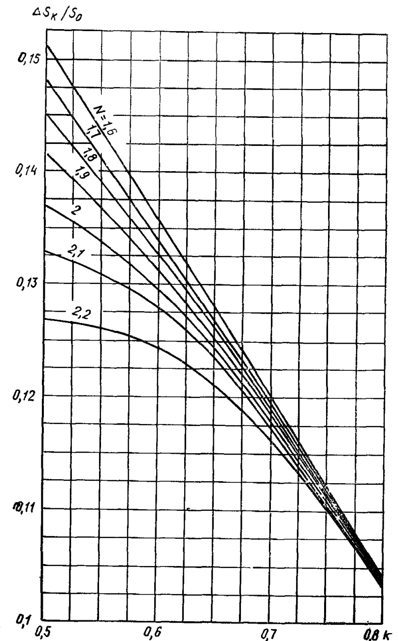
Рис. 2. График для определения относительной величины дополнительной осадки кормы судна \frac{\Delta S_K}{S_0} при входе (выходе) в камеру через верхнюю голову шлюза
