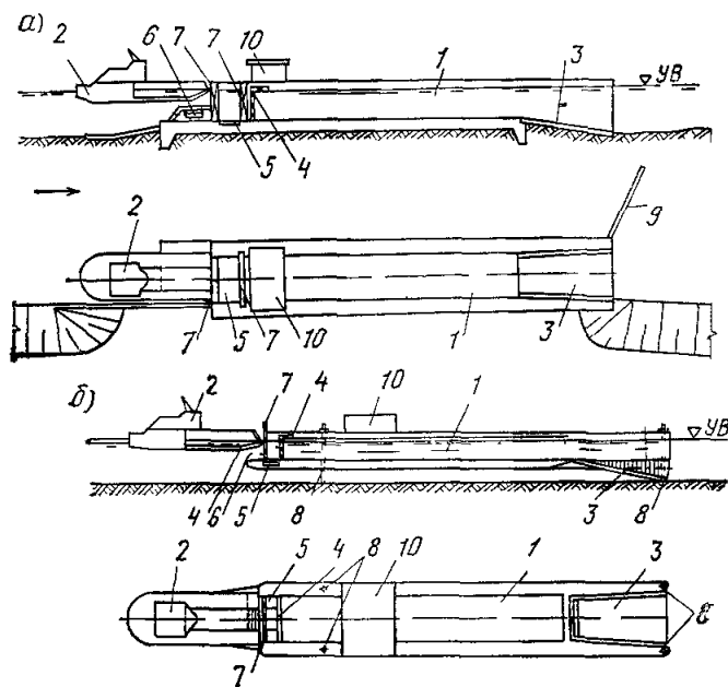
Рис. 13. Рыбонакопители (планы и разрезы)
