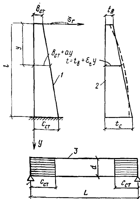
Рис. 1. Схема и определению свободных температурных деформаций элемента сооружения
