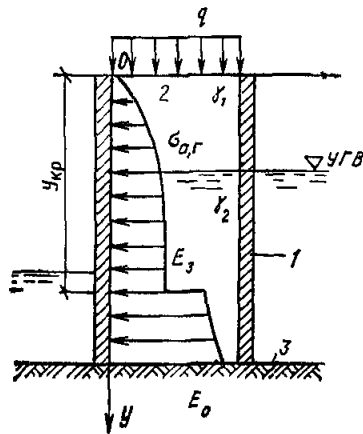
Рис. 2. Схема к расчету давления грунта на внутренние стены ячеек (оболочек)
