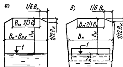
Рис. 3. Подмостовые габариты
